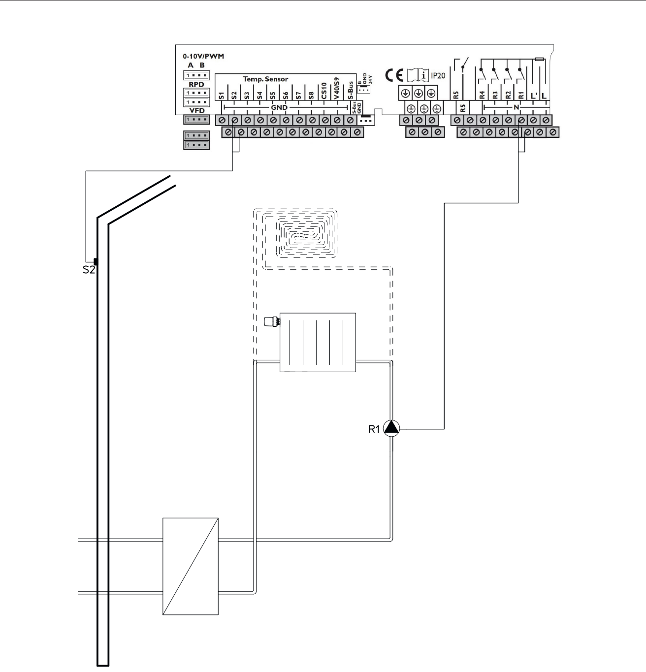
Fig. 52: Schéma 8, un circuit de chauffage direct
