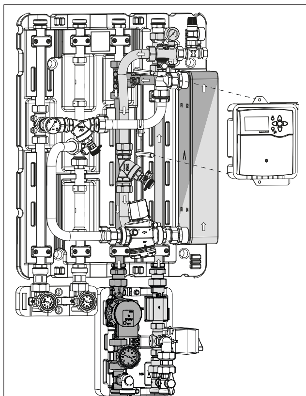
Fig. 21: Côté secondaire - Raccordement circuit de chauffage Regudis H-HT / Regudis H-MT (raccordement par le bas)
