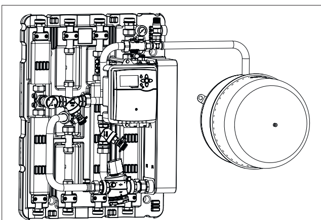
Fig. 39: Vase d'expansion à membrane monté
