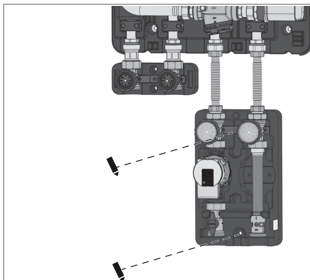
Fig. 31: Vissage du groupe avec circulateur (raccordement par le bas)
