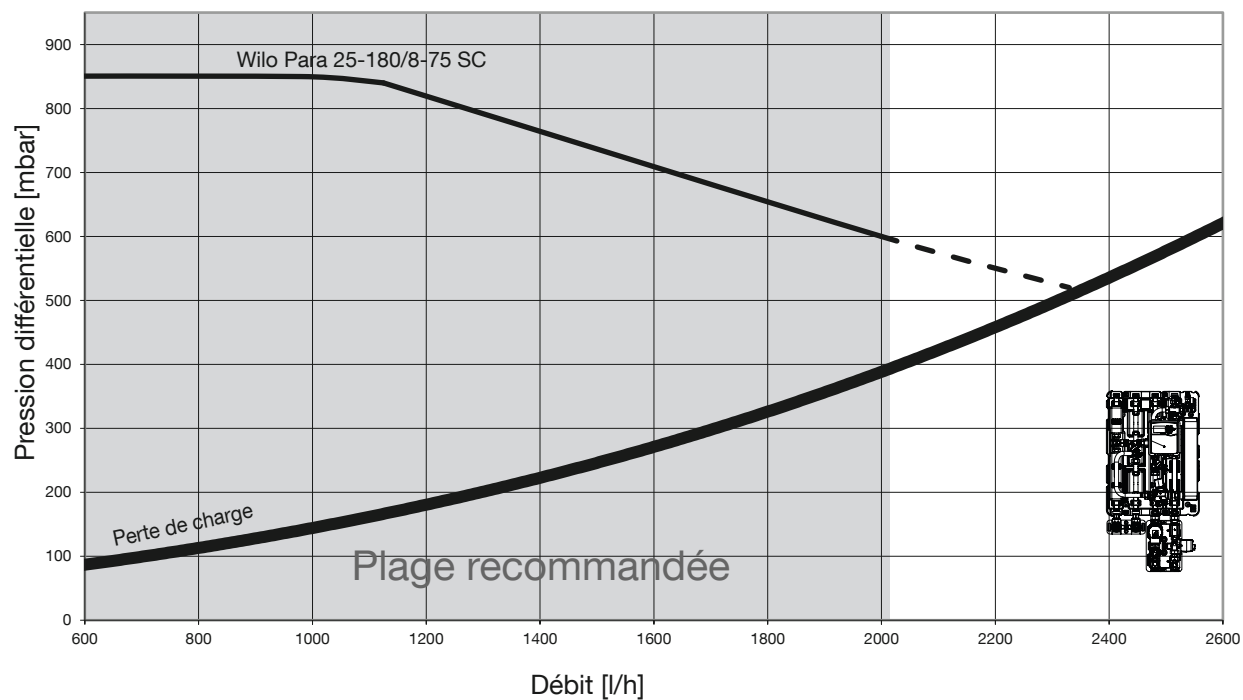
Fig. 59: Perte de charge circuit secondaire - Sous-station avec module de commutation HT
