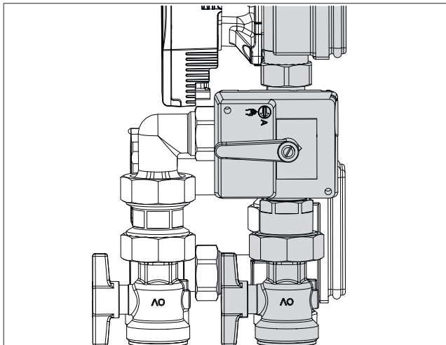
Fig. 19: Position du commutateur du robinet de commutation (service de chauffage)
