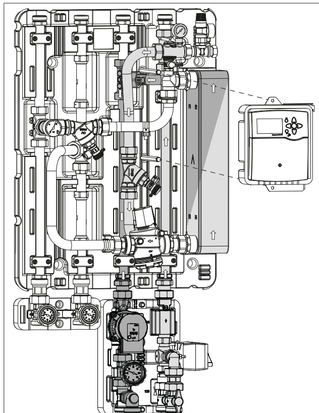
Fig. 22: Côté secondaire - Raccordement circuit ballon d'eau chaude Regudis H-HT / Regudis H-MT (raccordement par le bas)
