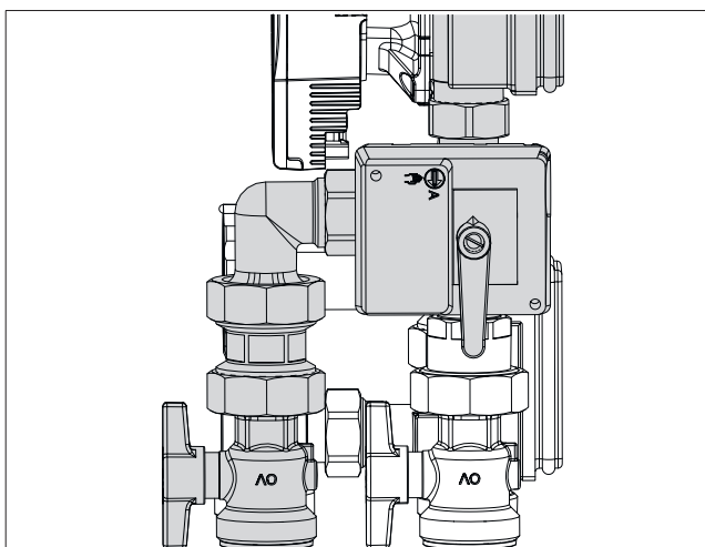
Fig. 20: Position du commutateur du robinet de commutation (réchauffage du ballon d'eau chaude)
