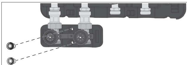
Fig. 28: Insertion des pièces d'écartement du jeu de raccordement avec robinets à tournant sphérique
