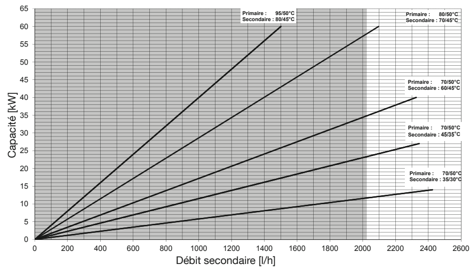
Fig. 63: Diagramme des puissances ; débit max. recommandé Regudis H en combinaison avec le module de commutation HT
