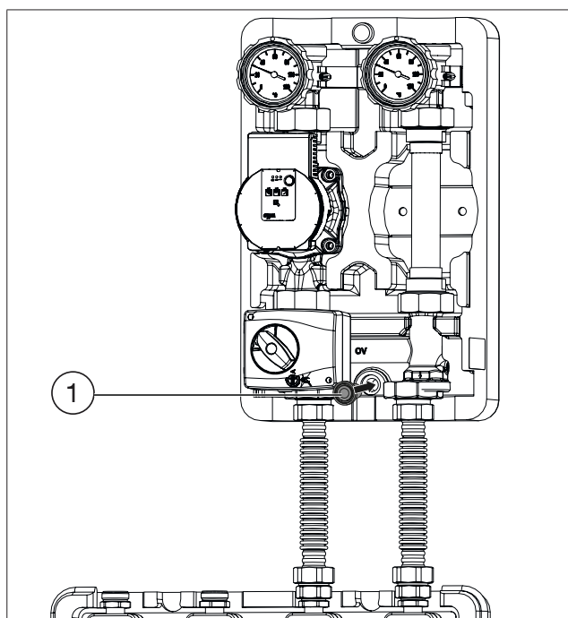
Fig. 36: Vissage du tube de raccordement (raccordement par le haut)
