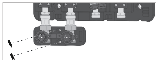
Fig. 27: Marquage des trous de perçage pour les vis de fixation
