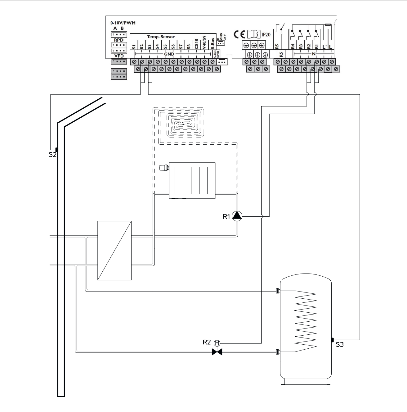
Fig. 48: Schéma 4, un circuit de chauffage direct, préparation d'E.C.S. directe
