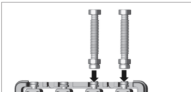
Fig. 36: Vissage du tube de raccordement (raccordement par le haut)
