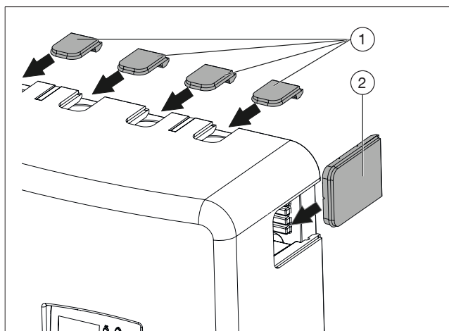
Fig. 40: Capots de protection dans l'isolation
