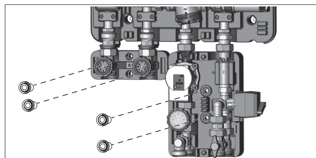
Fig. 34: Insertion des pièces d'écartement du module de commutation HT
