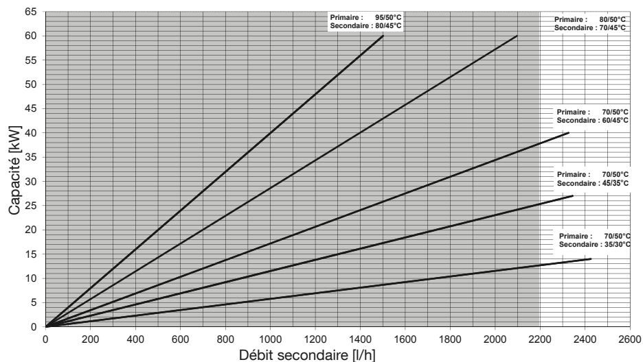
Fig. 65: Diagramme des puissances ; débit max. recommandé Regudis H en combinaison avec Regumat M3
