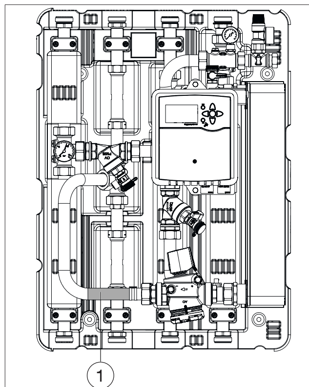
Fig. 41: Mise à la terre de la sous-station
