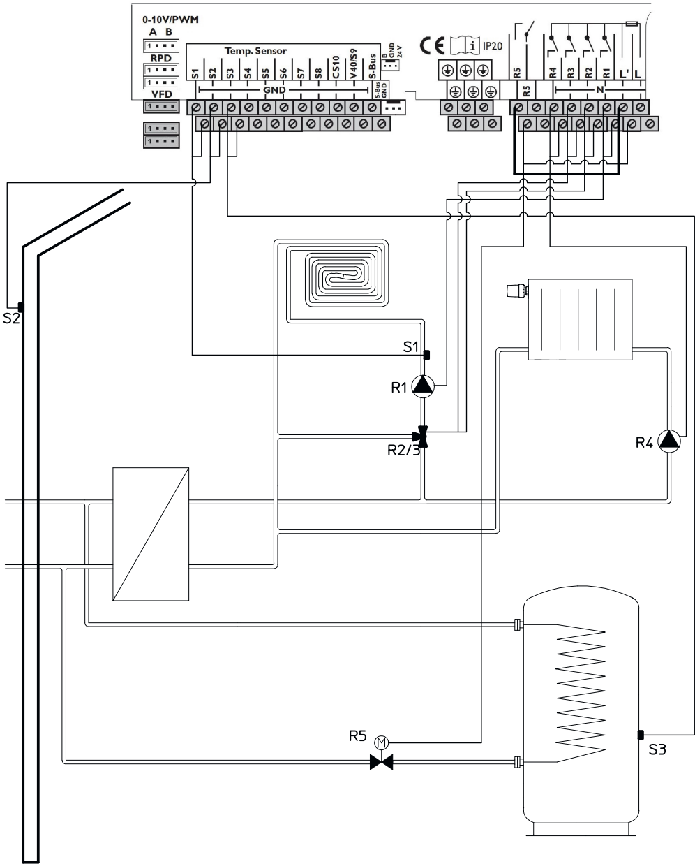
Fig. 50: Schéma 6, un circuit de chauffage mélangé et un circuit de chauffage direct, préparation d'E.C.S. directe
