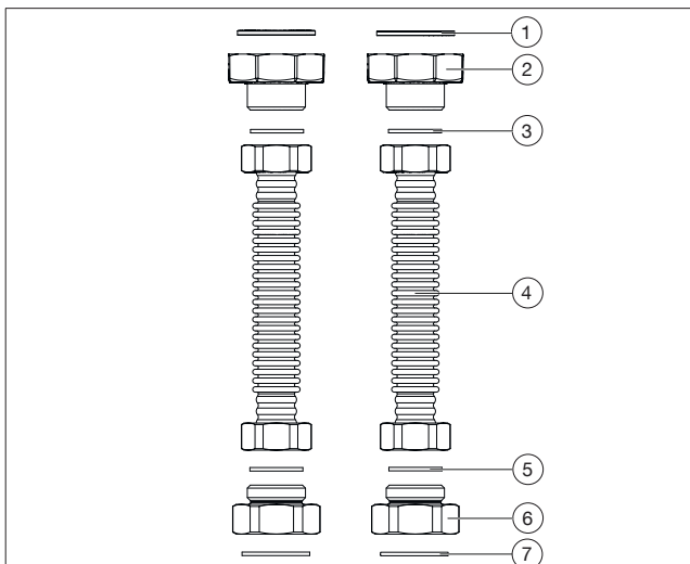
Fig. 35: Configuration du jeu de raccordement
