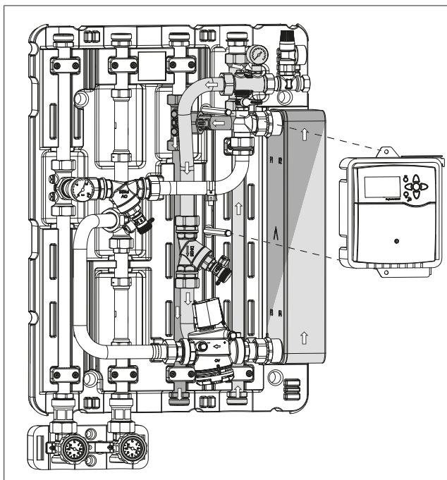
Fig. 17: Côté secondaire Regudis H-HT (exemple : raccordement par le bas)
