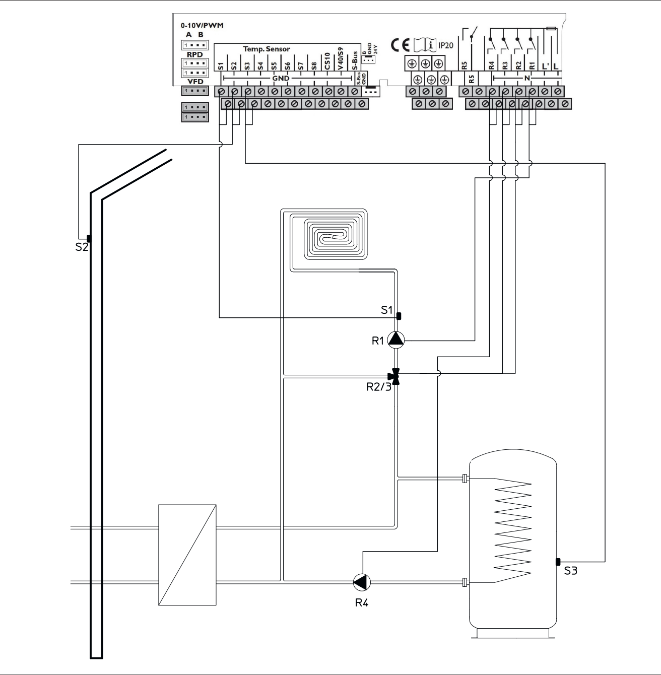
Fig. 46: Schéma 2, un circuit de chauffage mélangé, préparation d'E.C.S. indirecte
