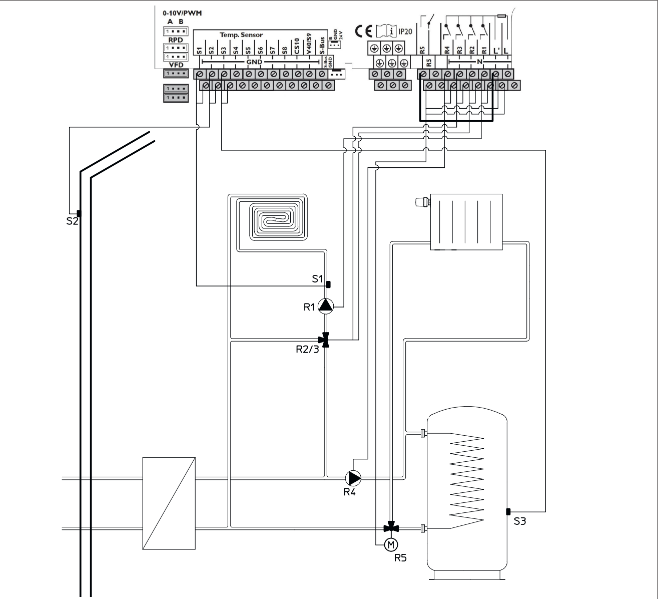
Fig. 54: Schéma 10, un circuit de chauffage mélangé et un circuit de chauffage direct, préparation d'E.C.S. indirecte
