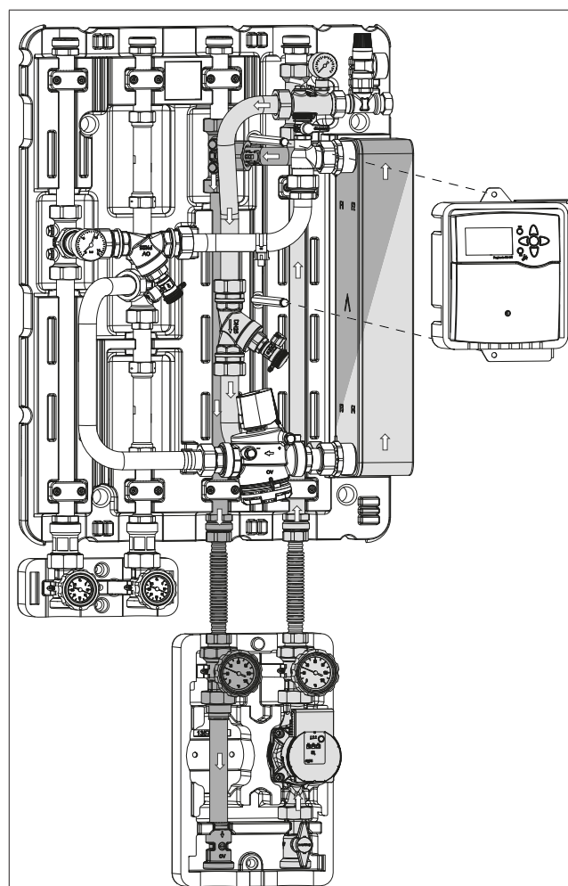
Fig. 18: Côté secondaire Regudis H-H / Regudis H-M (exemple : raccordement par le bas)
