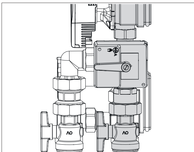
Fig. 23: Position du commutateur du robinet de commutation (service de chauffage)
