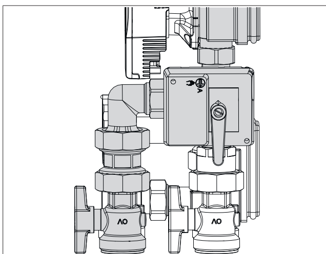
Fig. 24: Position du commutateur du robinet de commutation (réchauffage du ballon d'eau chaude)
