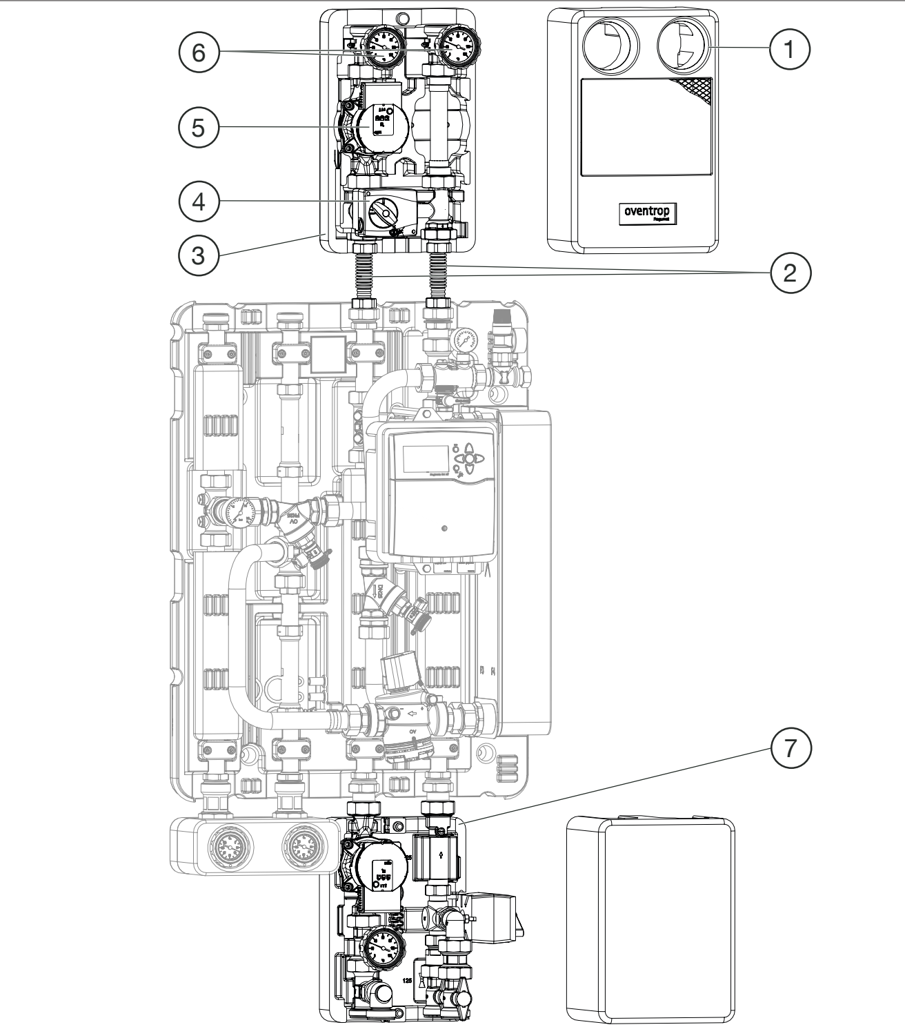
Fig. 13: Sous-station avec jeu de raccordement avec robinets à tournant sphérique, Regumat M3 et module de commutation HT
