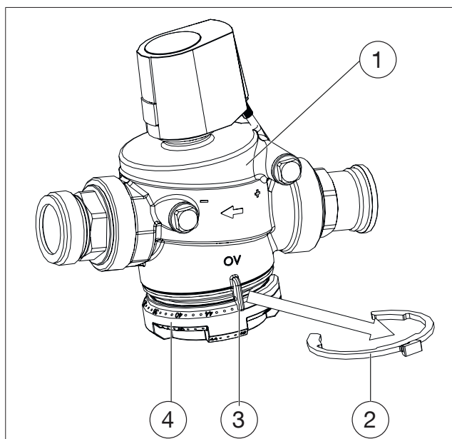
Fig. 42: Démontage du bague de blocage
