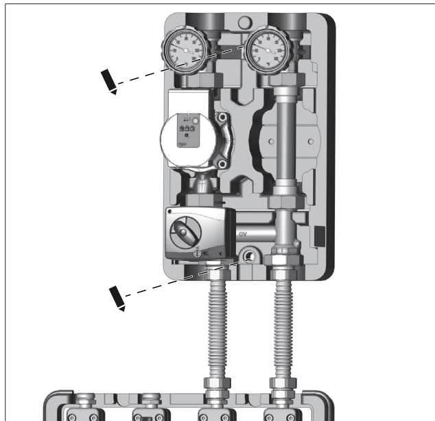
Fig. 37: Vissage du groupe avec circulateur (raccordement par le haut)
