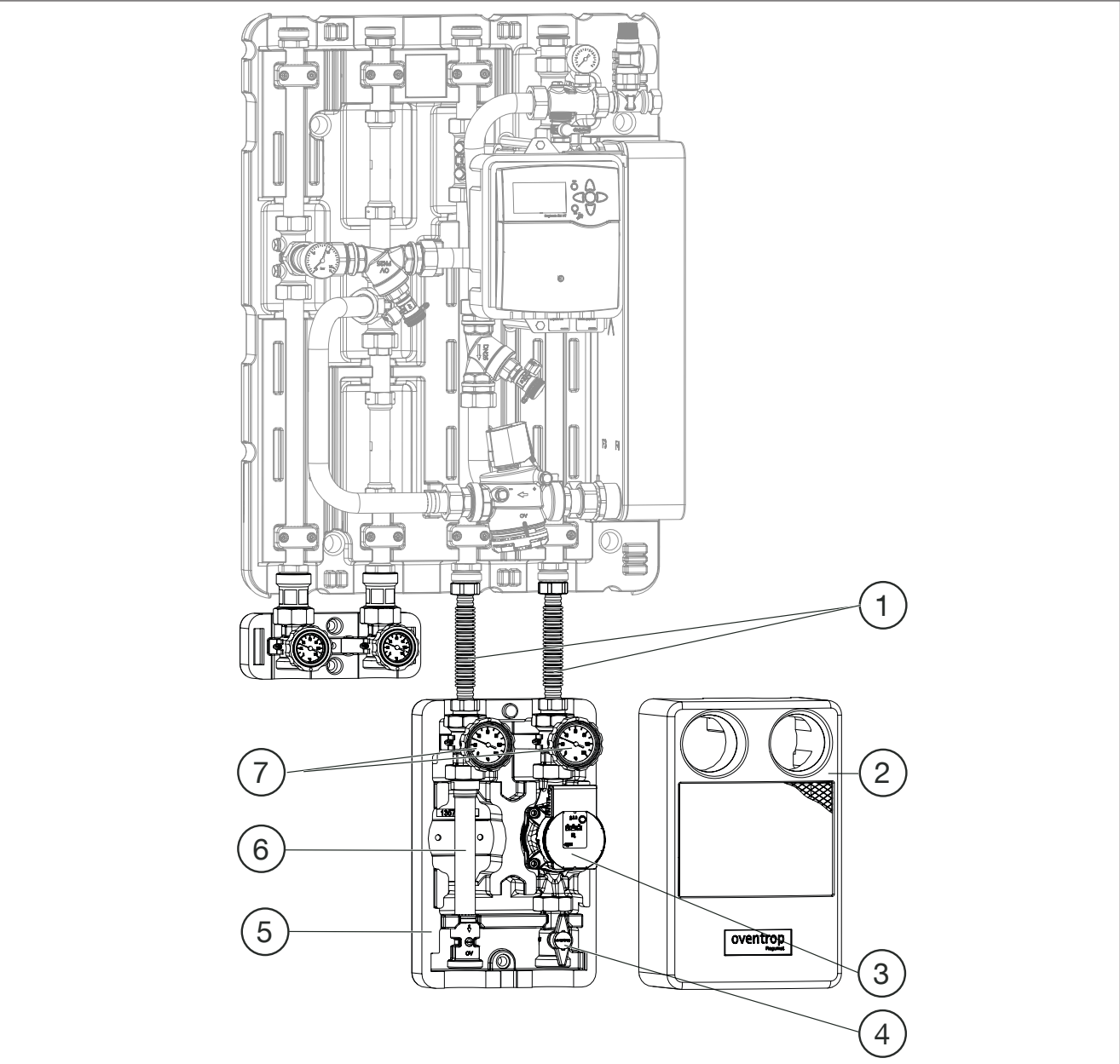
Fig. 9: Sous-station avec jeu de raccordement avec robinets à tournant sphérique et Regumat S
