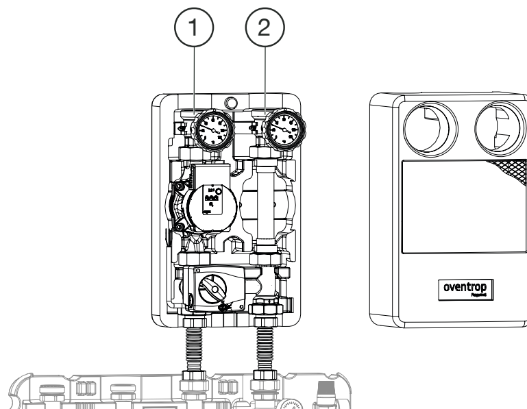
Fig. 14: Raccordements de la station Regudis H-MHT au Regumat M3 (service avec surface chauffante)
