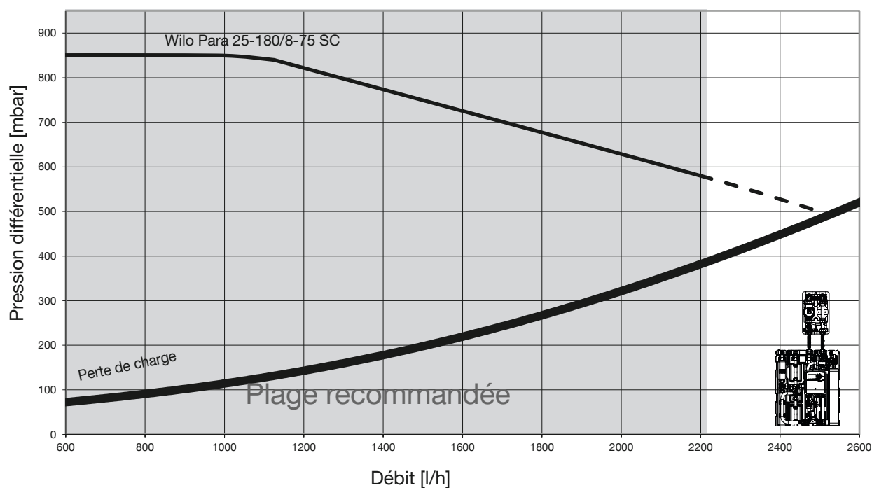
Fig. 58: Perte de charge circuit secondaire - Sous-station avec Regumat M3
