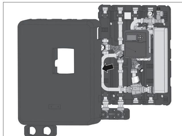
Fig. 26: Démontage des isolations avant
