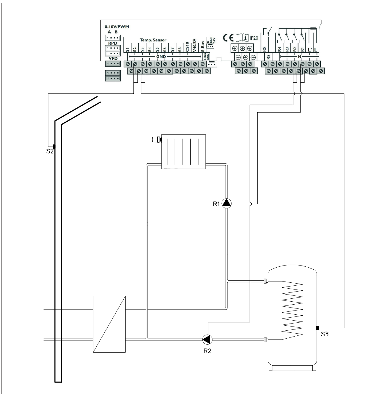
Fig. 45: Schéma 1, un circuit de chauffage direct, préparation d'E.C.S. indirecte
