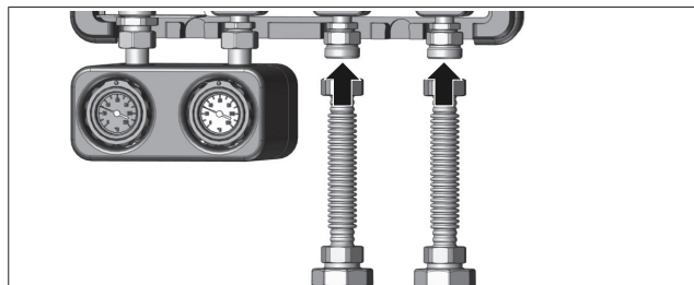
Fig. 30: Vissage du tube de raccordement (raccordement par le bas)
