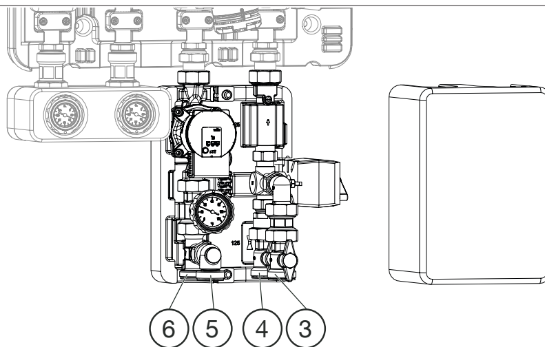
Fig. 15: Raccordements de la station Regudis H-MHT au module de raccordement HT (service avec radiateurs et réchauffage du ballon d'eau chaude)
