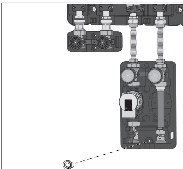
Fig. 32: Insertion de la pièce d'écartement du Regumat S
