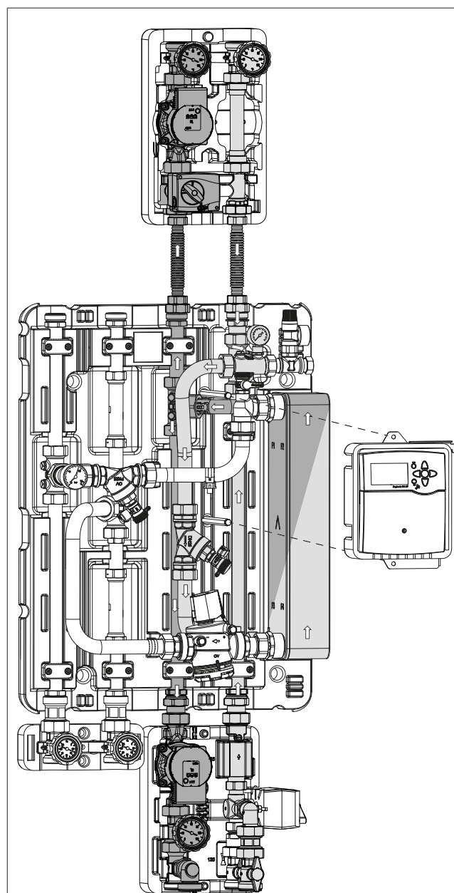
Fig. 25: Côte secondaire Regudis H-MHT (exemple réchauffage du ballon d'eau chaude)
