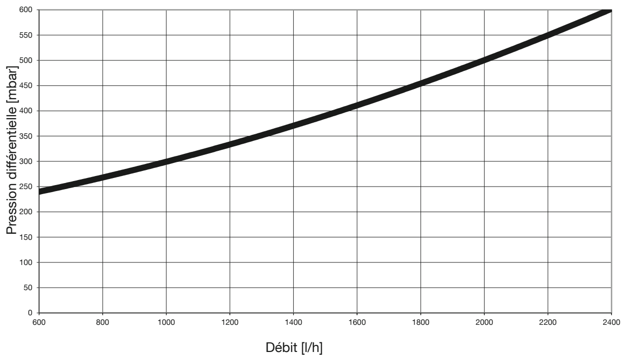
Fig. 55: Perte de charge circuit primaire Regudis H
