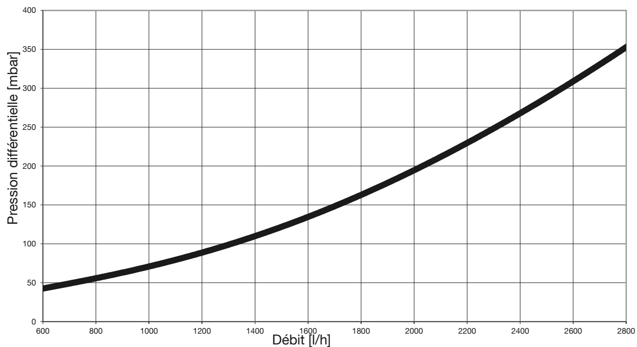
Fig. 56: Perte de charge circuit secondaire Regudis H
