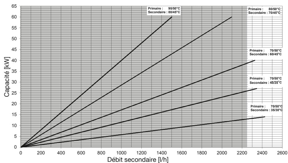
Fig. 64: Diagramme des puissances ; débit max. recommandé Regudis H en combinaison avec Regumat S
