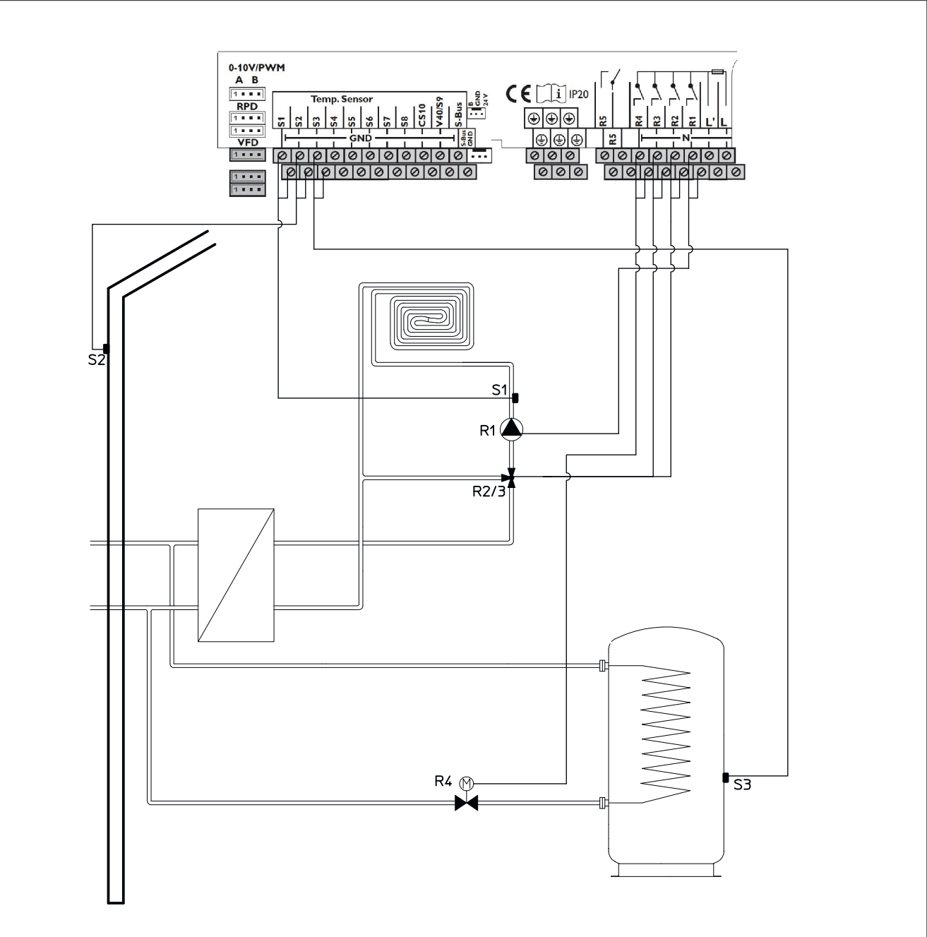
Fig. 49: Schéma 5, un circuit de chauffage mélangé, préparation d'E.C.S. directe
