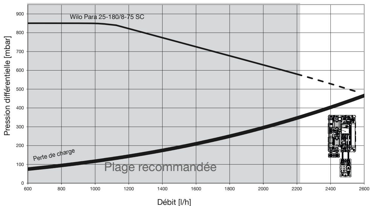
Fig. 57: Perte de charge circuit secondaire - Sous-station avec Regumat S
