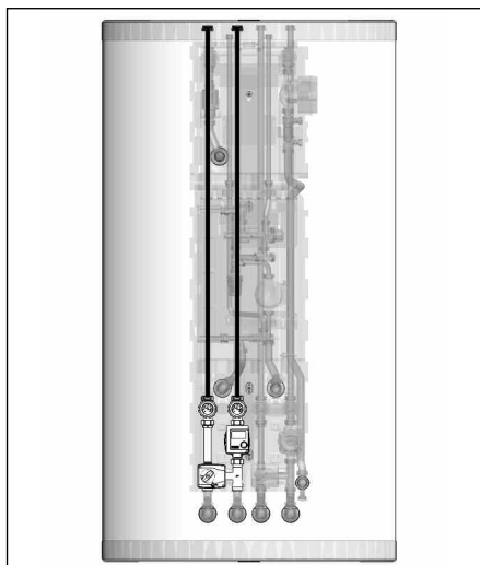
Fig. 1.2 Schéma de montage pour jeu d'extension (réf.: 138 35 81)
