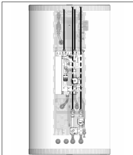
Fig. 1.1 Schema d'installazione per il set di collegamento (Codice n.: 138 35 80)
