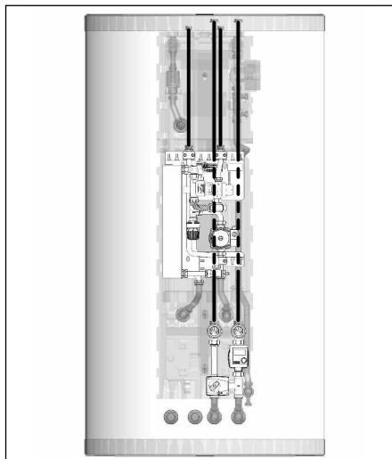
Abb. 1.1 Montageschema für Anschluss-Set (Art.-Nr.: 138 35 80)
