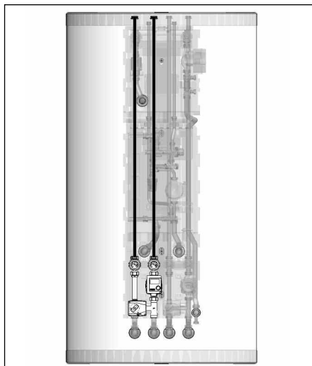
Abb. 1.2 Montageschema für Anschluss-Set- erweiterung (Art.-Nr.: 138 35 81)
