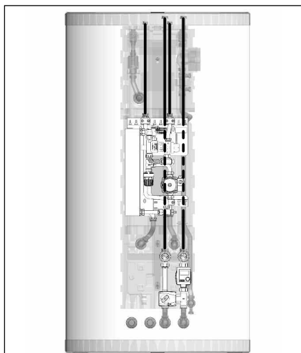
Fig. 1.1 Schéma de montage pour jeu de raccordement (réf.: 138 35 80)
