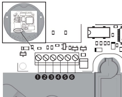
Bornes del Datalog CS-BS-1
