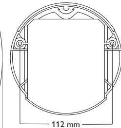
Posición de los orificios de fijación
