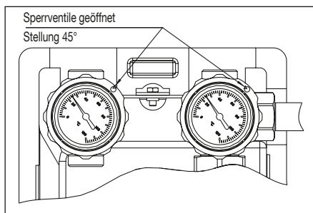
Abb. 4.4 Sperrventile geöffnet
