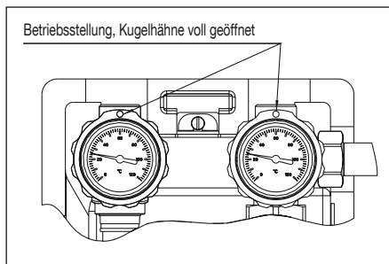
Abb. 4.3 Betriebsstellung
