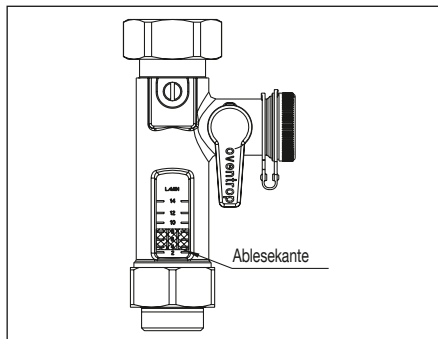
Abb. 4.5 Abgleichventil
