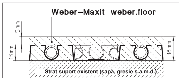
Weber-Maxit weber.floor (strat minim de acoperire 5 mm, înălțime constructivă totală 18 mm)
