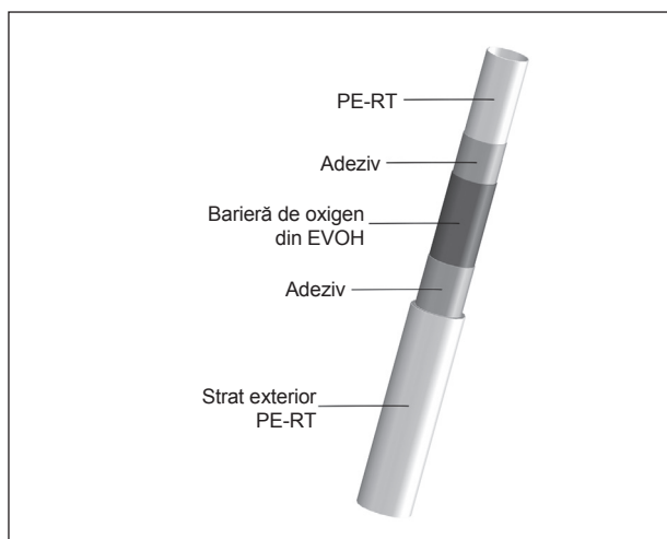
Țevă din plastic PE-RT „Copert“ 12 x 2 mm
