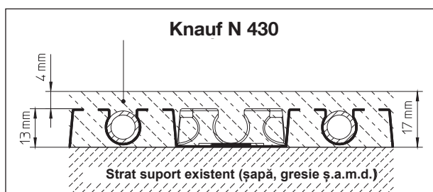
Knauf N 430 (strat minim de acoperire 4 mm, înălțime constructivă totală 17 mm)
