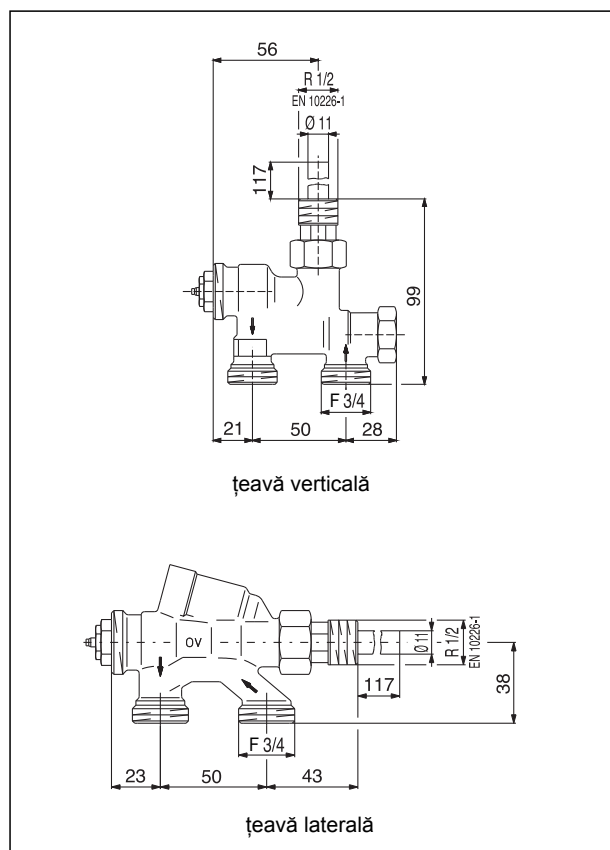
Dimensiuni ventile cu țeavă imersibilă (sisteme mono-/bitubulare)
