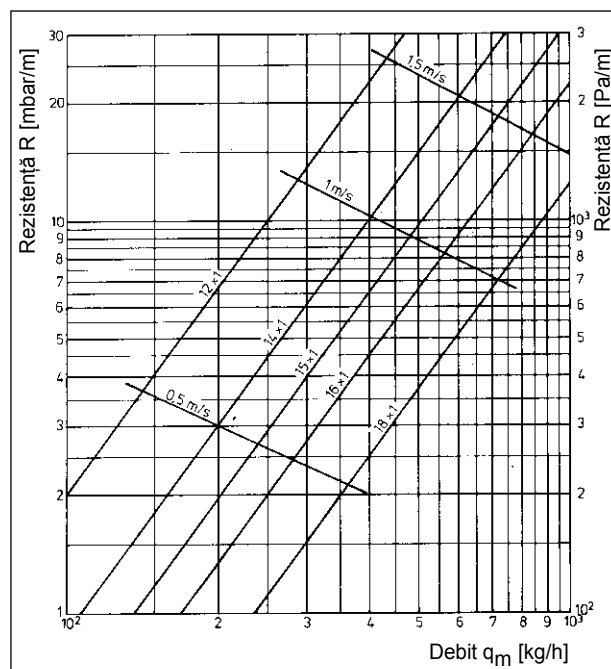
Diagrama 14 Țeavă din cupru Rezistență R în mbar/m
