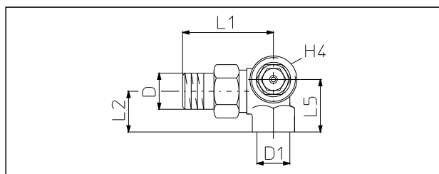
Dimensiuni ventil colțar în 3 axe, model cu racord pe dreapta
