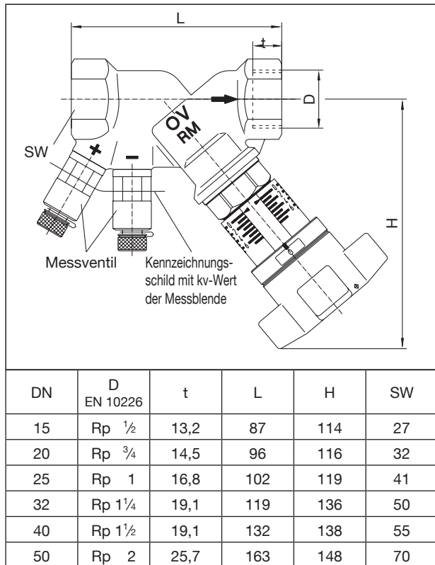
Maße „Hydrocontrol MTR“
