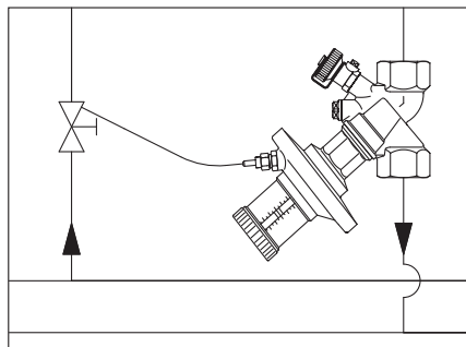
Exemplu: Reglarea presiunii diferențiale în instalații cu robineti termostatați thermostatic radiator valves (circuite cu debit mediu sau maxim)
