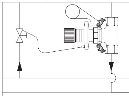
Exemplu: Reglarea presiunii diferențiale în instalații cu robineti termostatați (circuite cu debit scăzut sau mediu)
