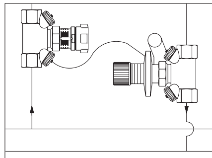
Exemplu: Reglarea presiunii diferențiale în instalații cu limitatori de debit și cu robineti termostatați presetati
