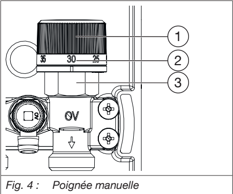
Fig. 4 : Poignée manuelle
