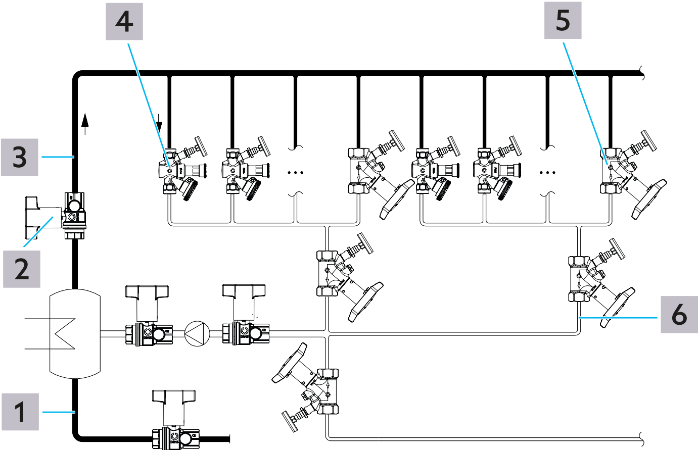
Ryc. 4: Schemat instalacji
