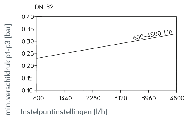
Afb. 13: Minimale verschildrukken
