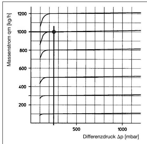
Ausschnitt aus Diagramm DN 20
