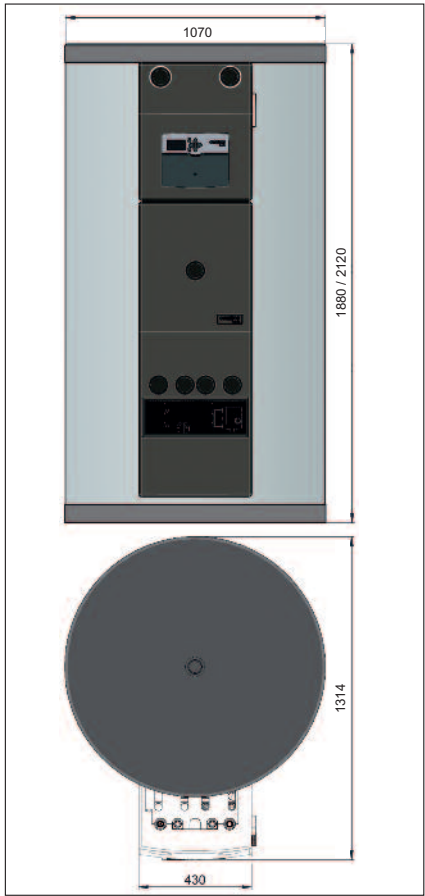
1-3 Dimensioni e dati tecnici sistema d'accumulo „Regucor WHS“.
