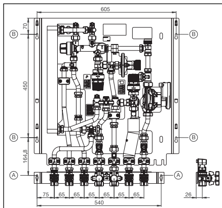
Abb. 6.2 Anschlusschema Kugelhahnanschlussleiste
