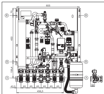
Abb. 6.1 Anschlusschema Kugelhahnanschlussleiste
