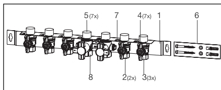
Abb. 3.1 „Regudis W“ Anschluss-Set
