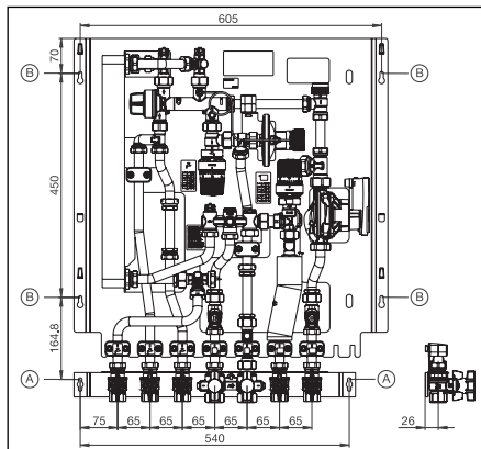
Fig. 6.2 Schéma de raccordement bloc de raccordement avec robinets à tournant sphérique
