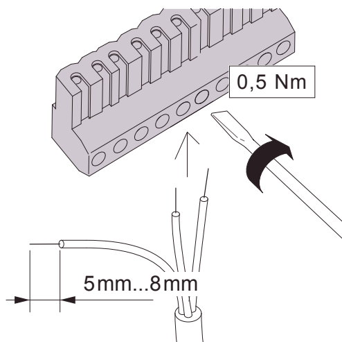
Abb. 20: Anschlusstecker verkabeln
