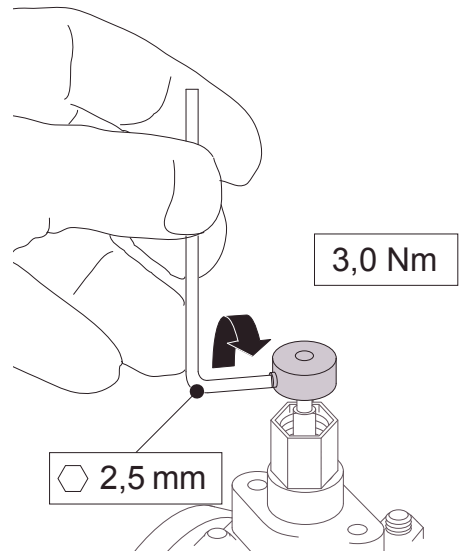
Abb. 7: Mitnehmerring positionieren
