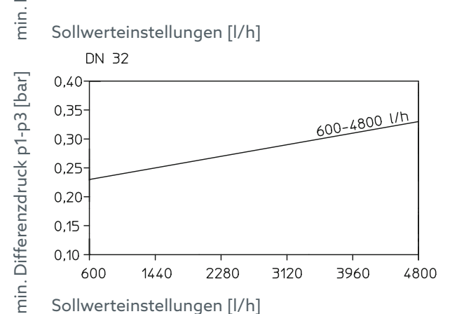
Abb. 13: Mindest-Differenzdrücke
