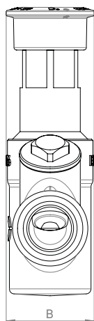
Fig. 3: Dimensiones frontales
