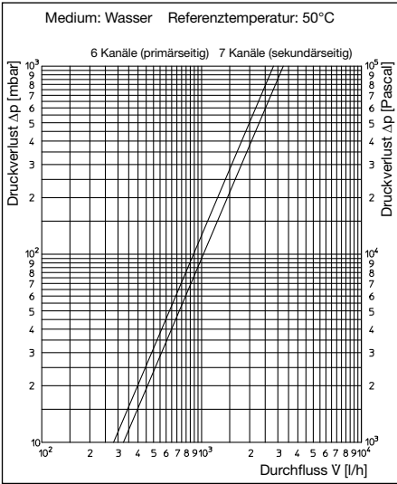
Abb. 7.2: Wärmeübertrager
