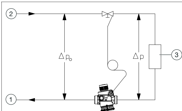
Abb. 4: Einbaubeispiel
