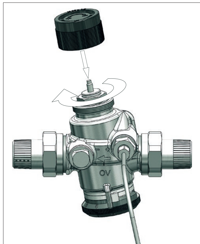
Abb. 5: Absperren
