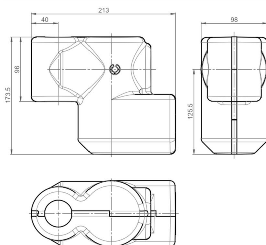
Für DN20 und DN25, vertikale Einbaulage (Art.-Nr. 1124191)
