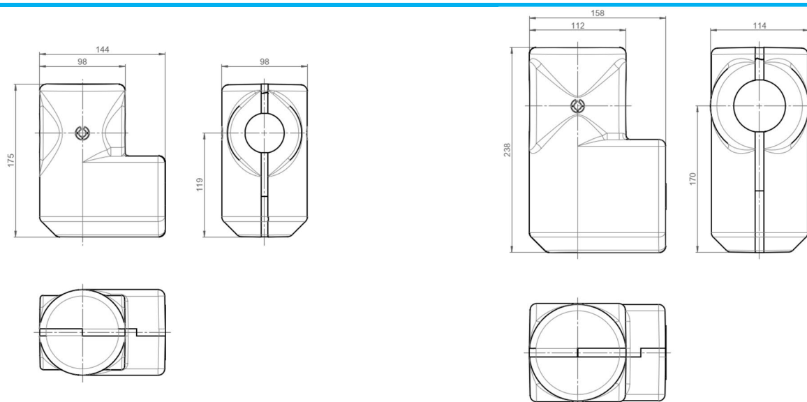
Für DN20 und DN25, horizontale Einbaulage (Art.-Nr. 1124091)
