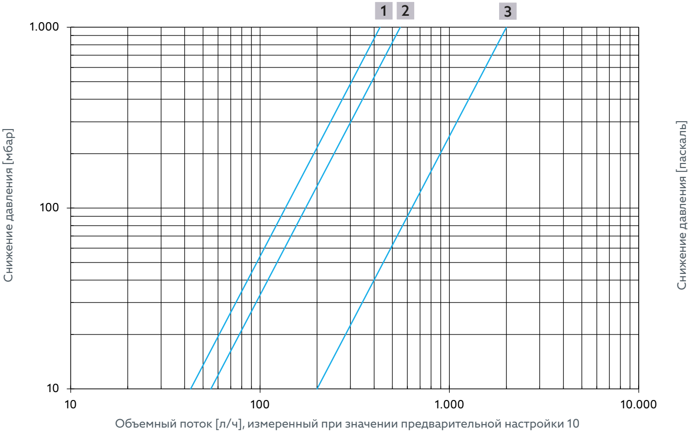
Рис. 20: Объемный поток Термическое регулирование для арт. № 4202554 и 4202754
