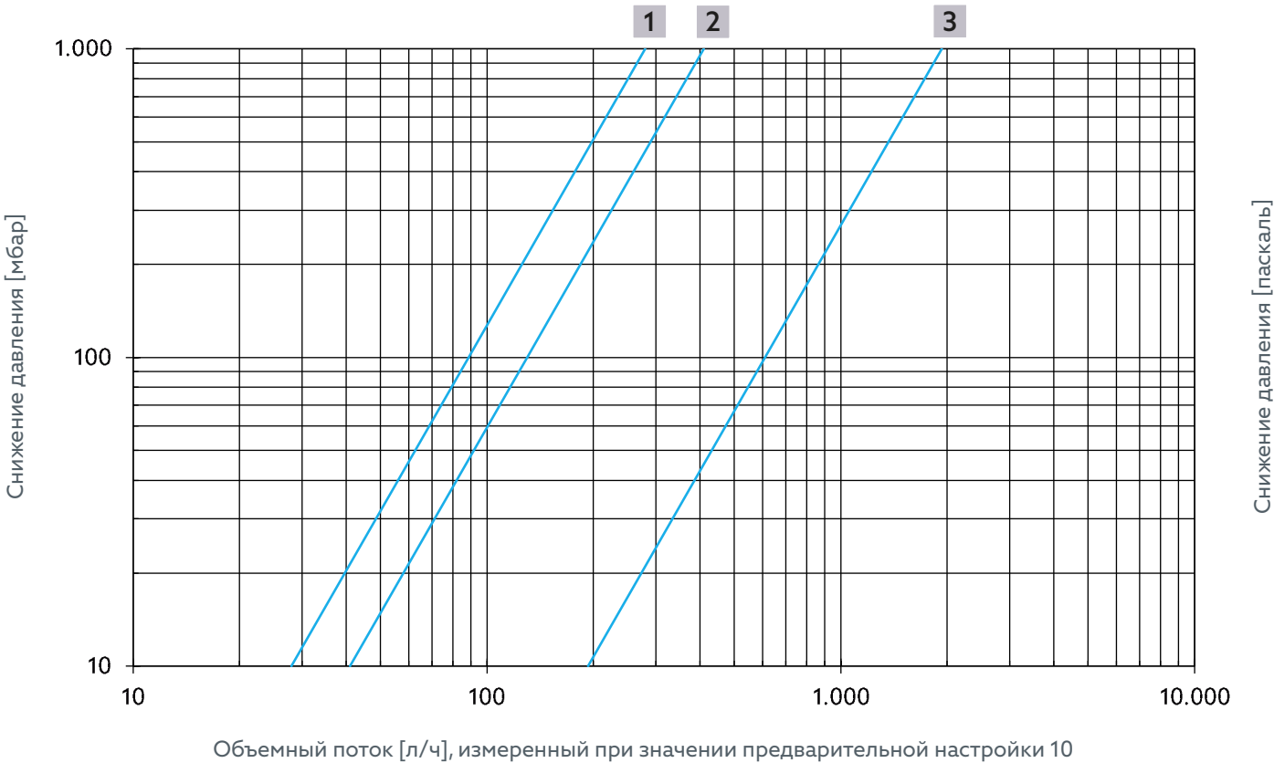
Рис. 19: Объемный поток Термическое регулирование для арт. № 4202506 и 4202706
