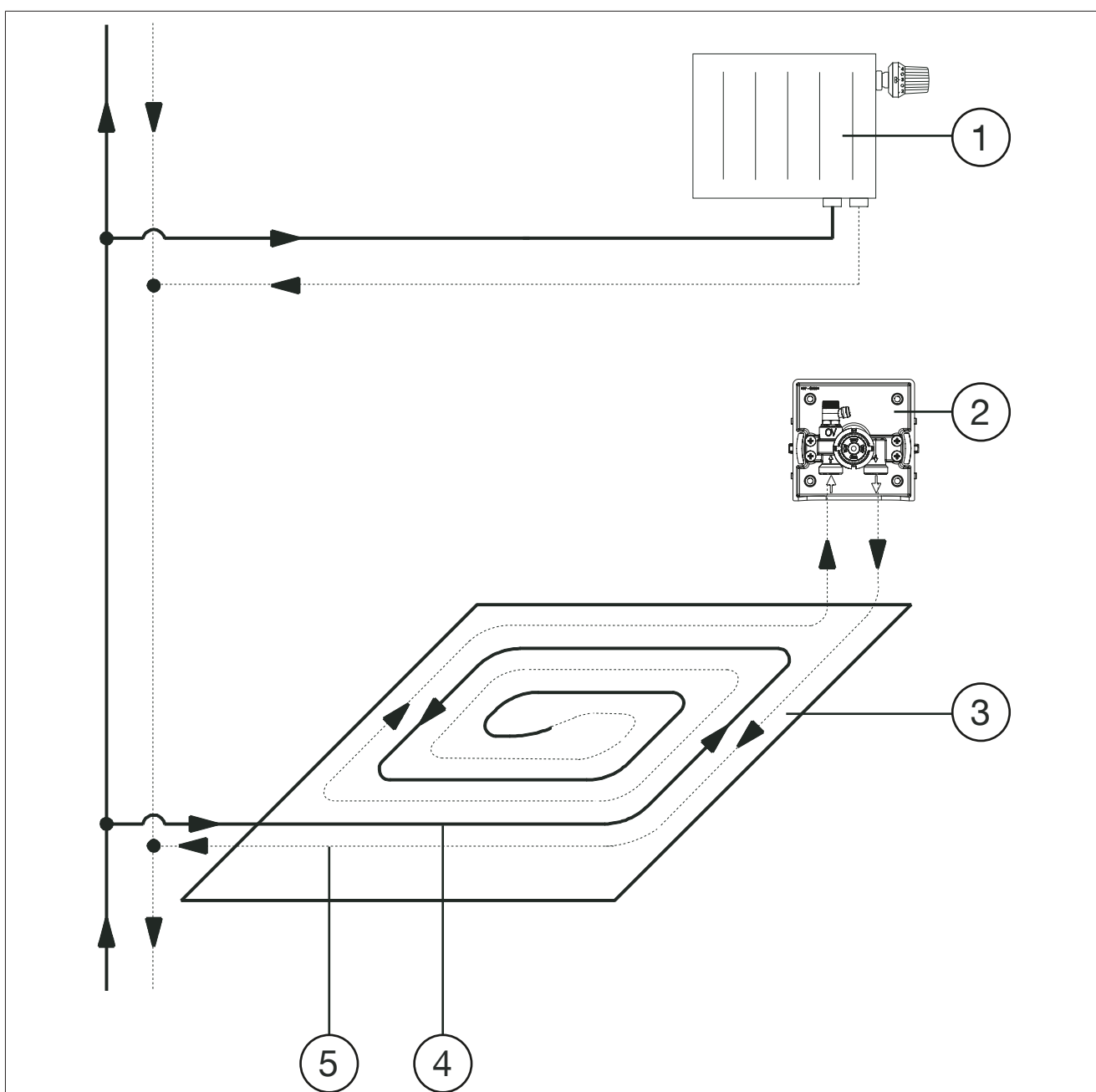
Fig. 1: Raccordement
