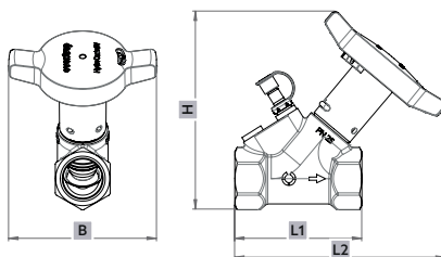
Abb. 2: Encombrenments vue de côté / vue de face - Version avec filetage
