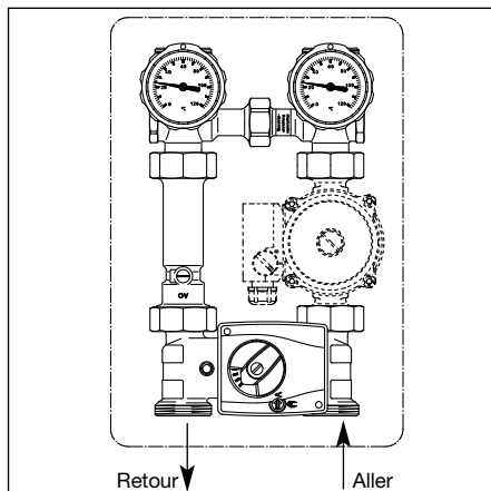
Exemple d'installation «Regumat M4»
