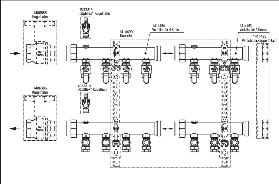
Abb. 10.1: Systemkomponenten
