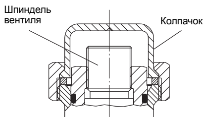
Рис. 7.1: Регулирующий вентиль
