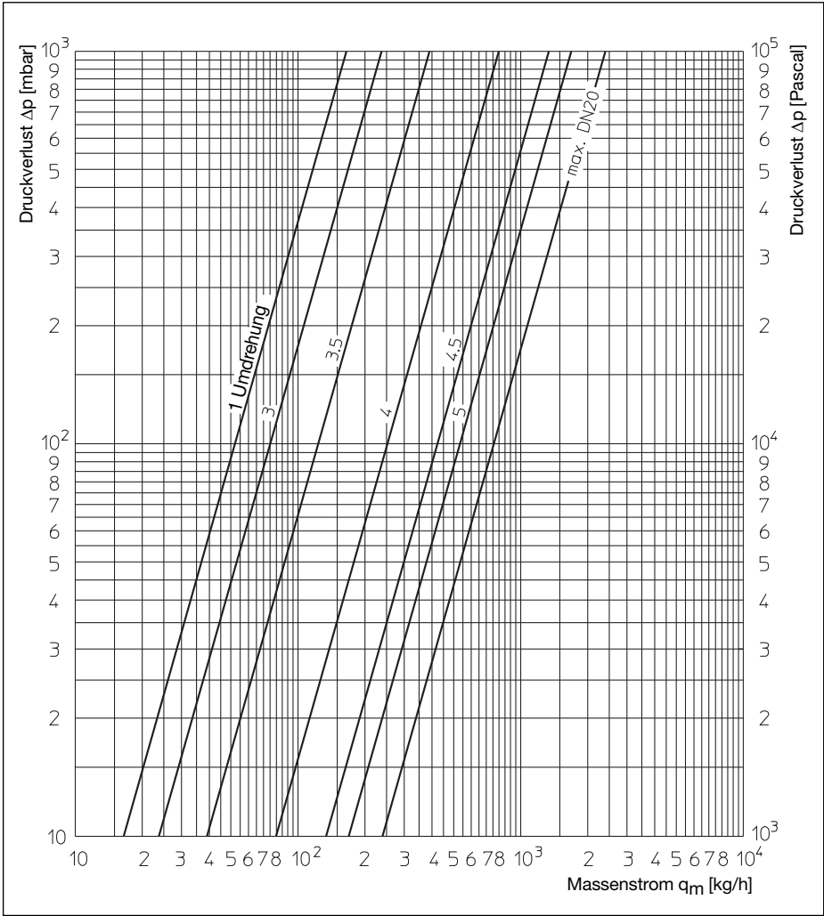
Abb. 9.1: Diagramm Reguliereinsatz für verschiedene Voreinstellungen
