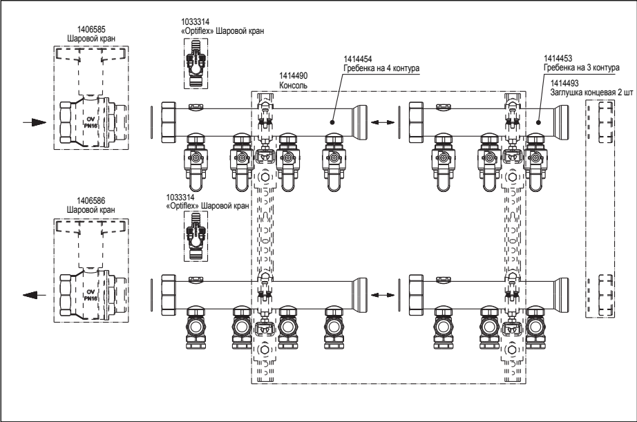
Рис. 10.1: Системные компоненты
