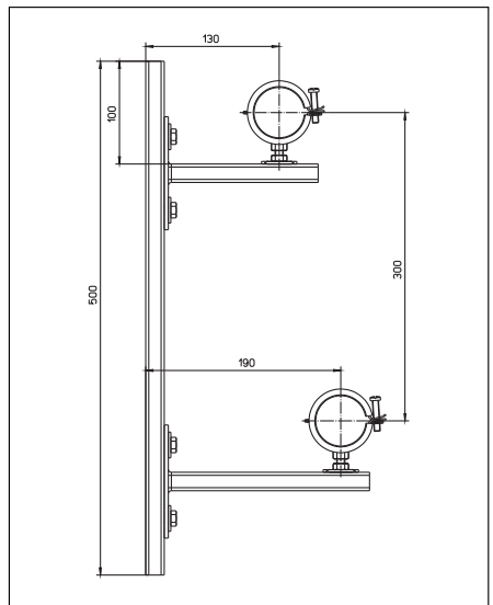
Abb. 5.2: Abmessungen Konsole
