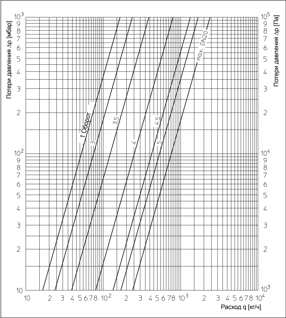
Рис. 9.1: Диаграмма настроек регулирующего вентиля
