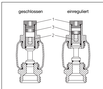
Abb. 3: Reguliereinsatz
