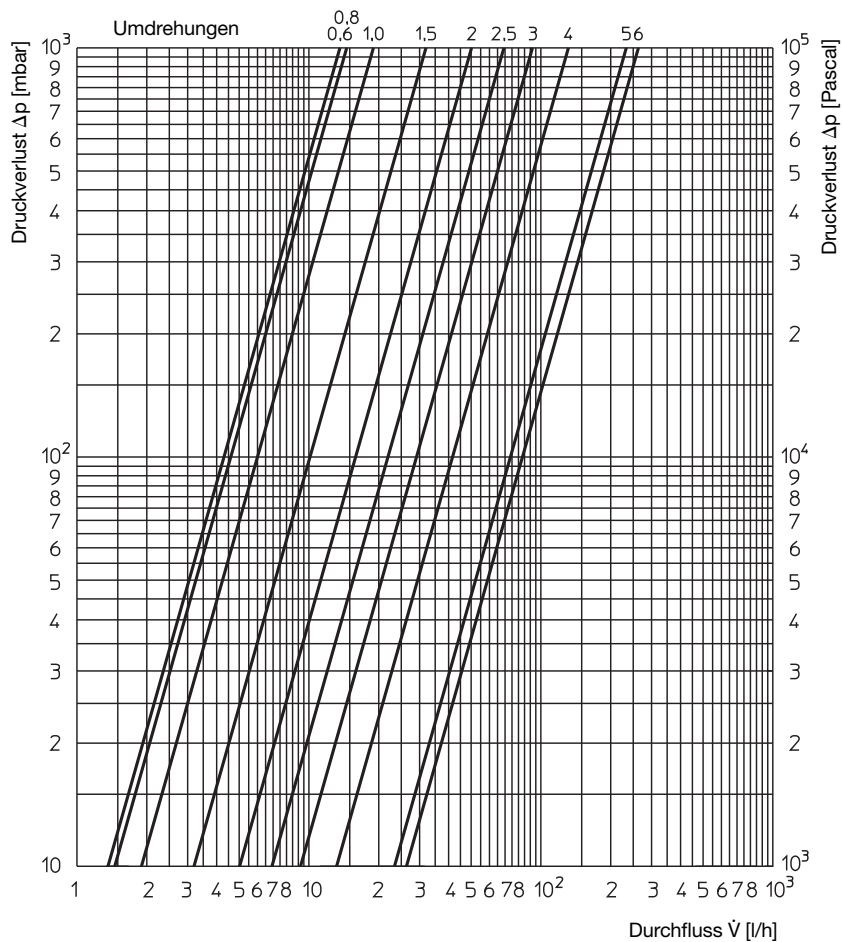
Diagramm 2: Druckverlustrdiagramm Bypass, bei geschlossenem Ventil
