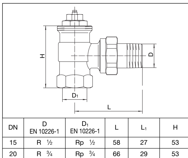
Dimensiuni ventil colțar
