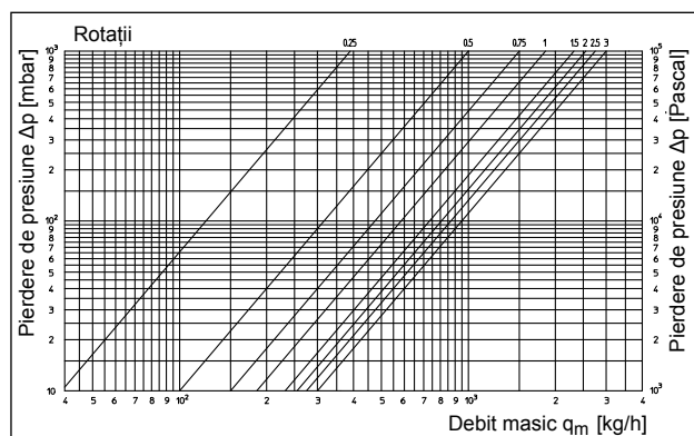
DN 15/20 model colțar și DN 25 model drept
