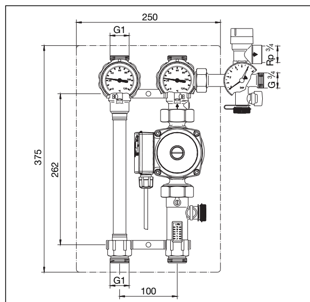
Station intermédiaire «Regusol-130»
