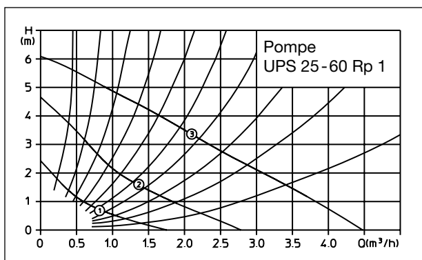
Courbes caractéristiques de la pompe:
