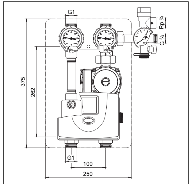
Station intermédiaire «Regusol EL-130»
