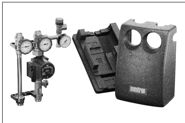
Station intermédiaire «Regusol-130»
