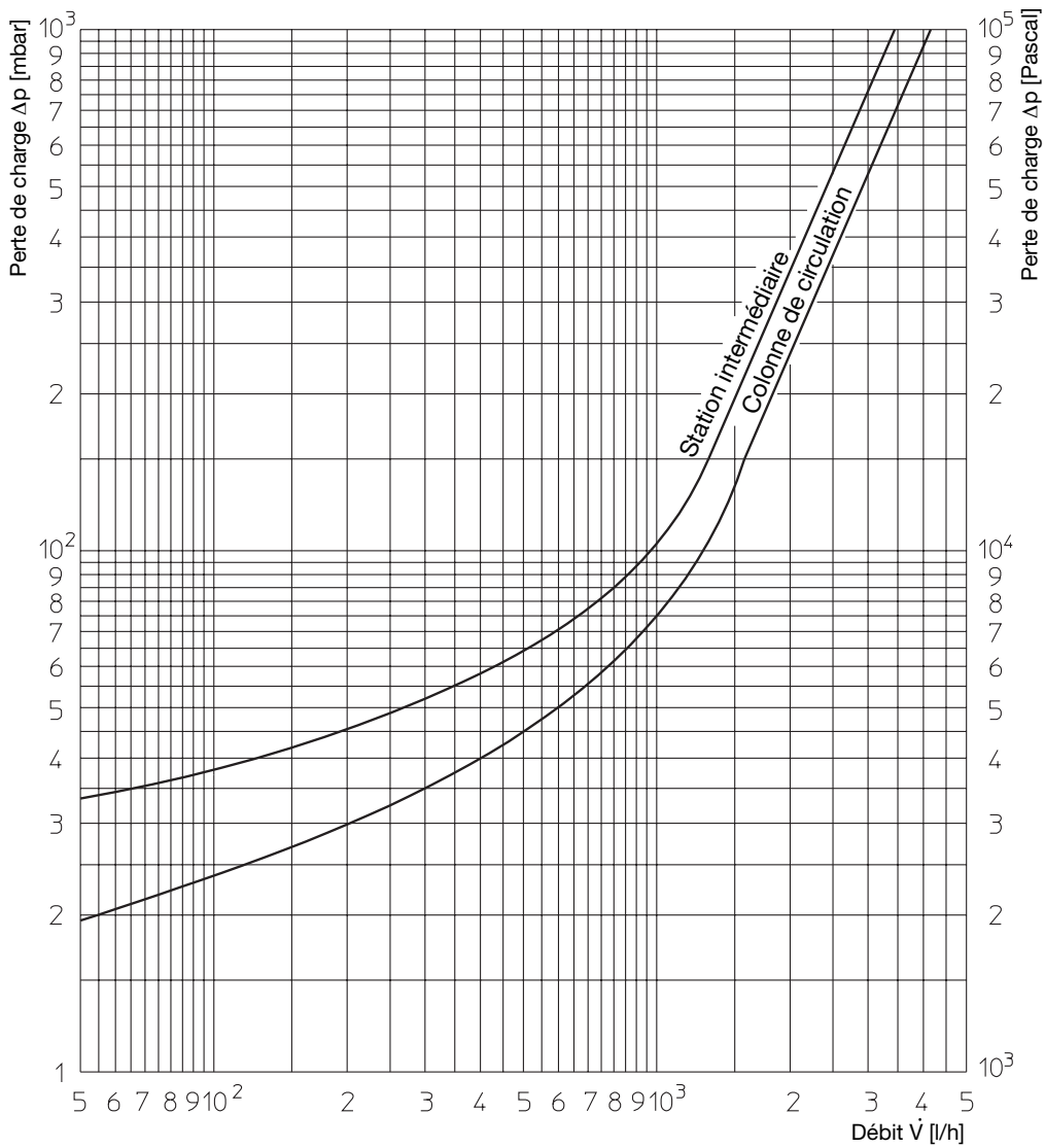
Courbes caractéristiques de la pompe:
