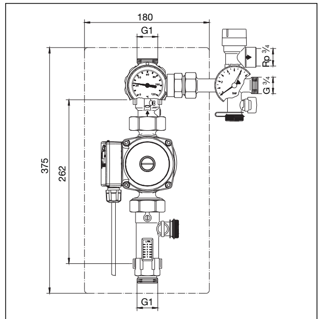
Colonne de circulation «Regusol-130»
