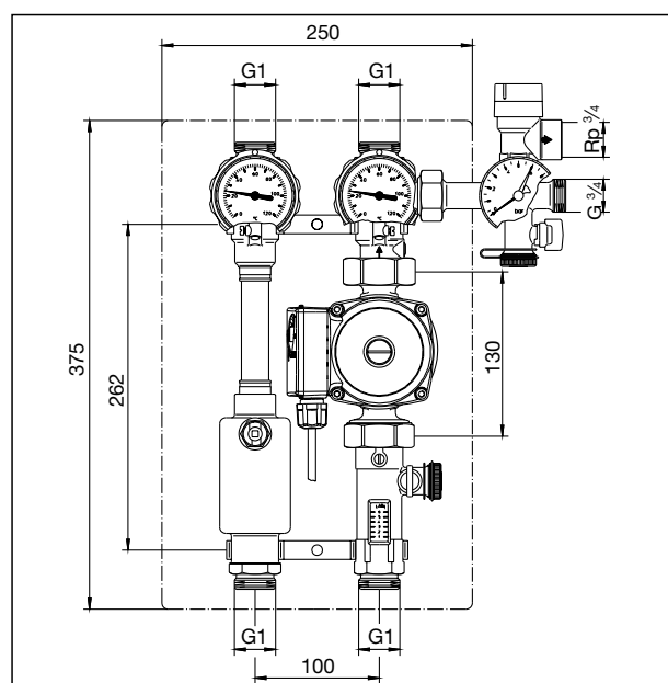
Station intermédiaire «Regusol L-130»
