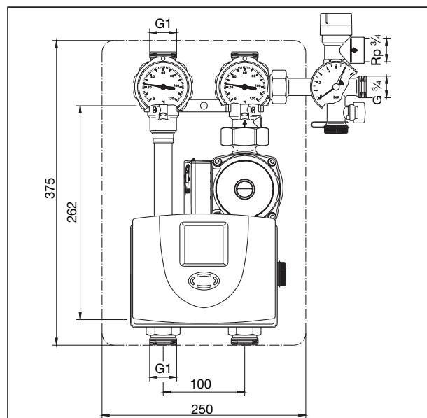
Station intermédiaire «Regusol E-130»
