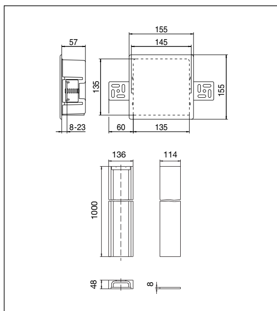
Maten „Unibox E RTL” en leidinginbouwkast
