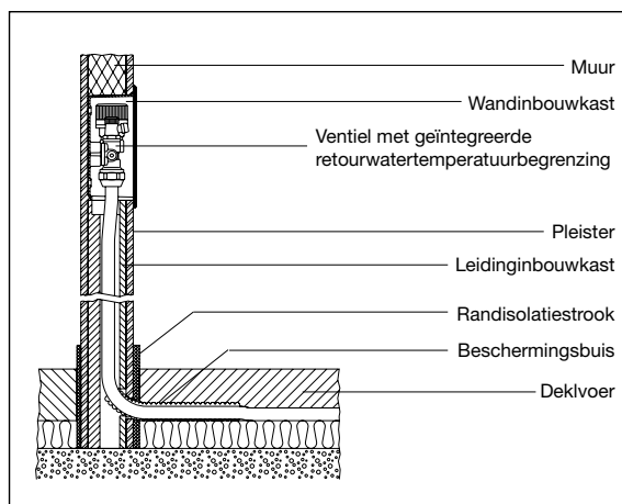
„Unibox E RTL”, inbouwdiepte 57 mm
