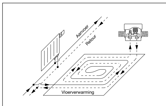
Inbouwschema retourwatertemperatuurbegrenzing
