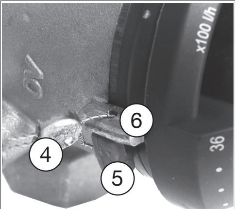
Fig. 12: Protection du préréglage
