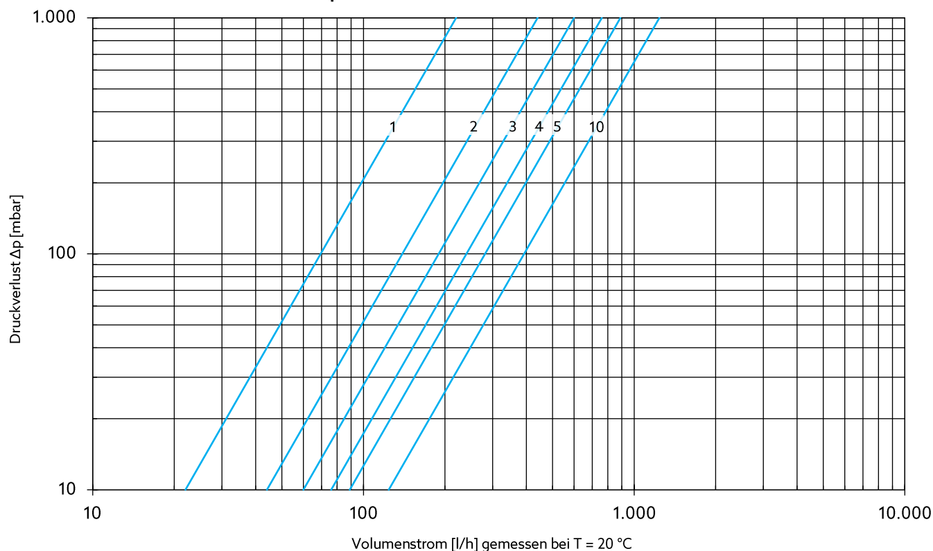
Volumenstrom Voreinstellwerte Aquastrom TV DN 15
