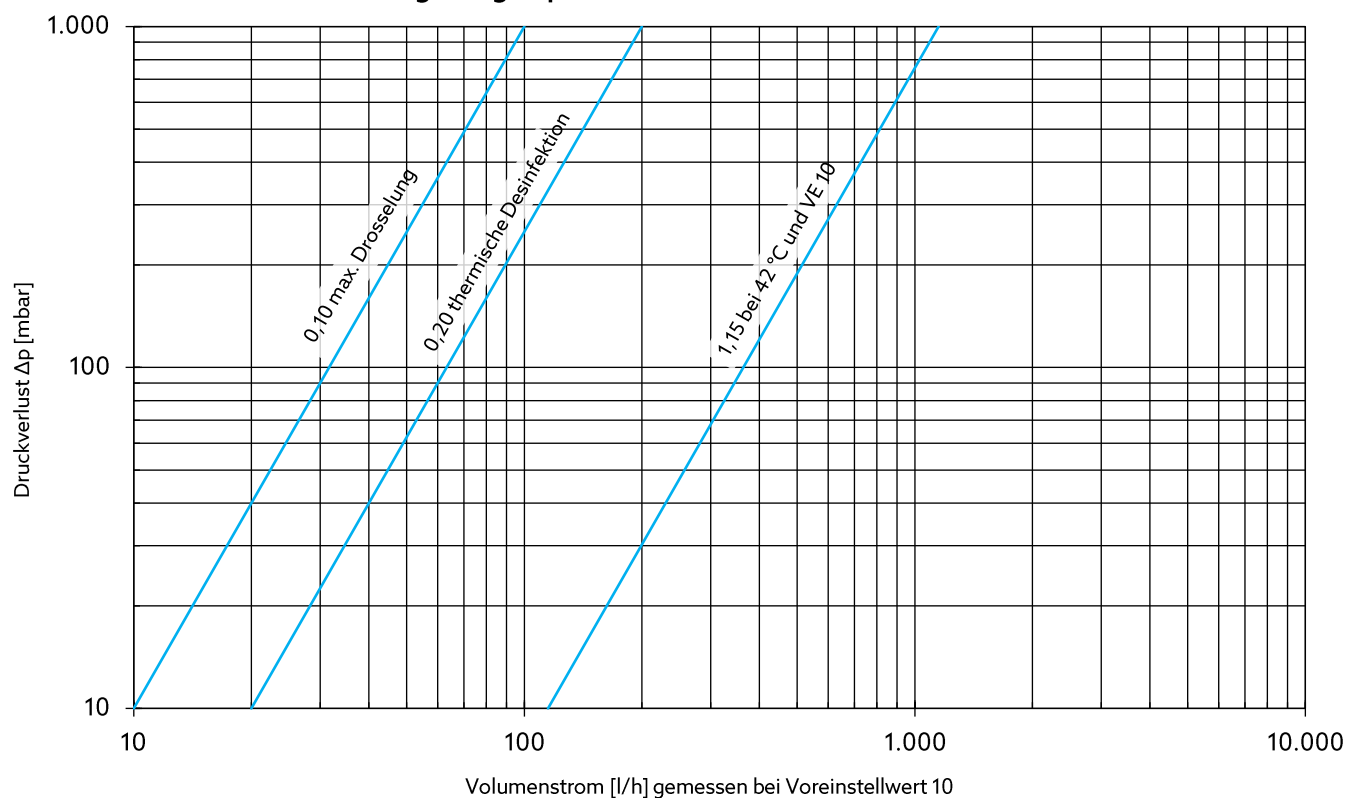
Volumenstrom Thermische Regelung Aquastrom TV DN 15
