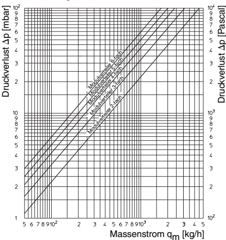
Modulverteiler für 3 Heizkreise
