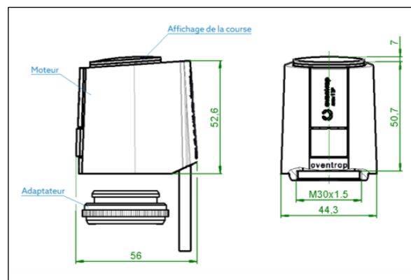
Encombres moteur avec interrupteur auxiliaire
