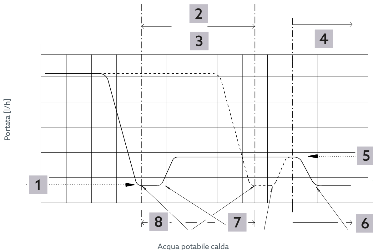
Fig. 6 - Regolazione termica
