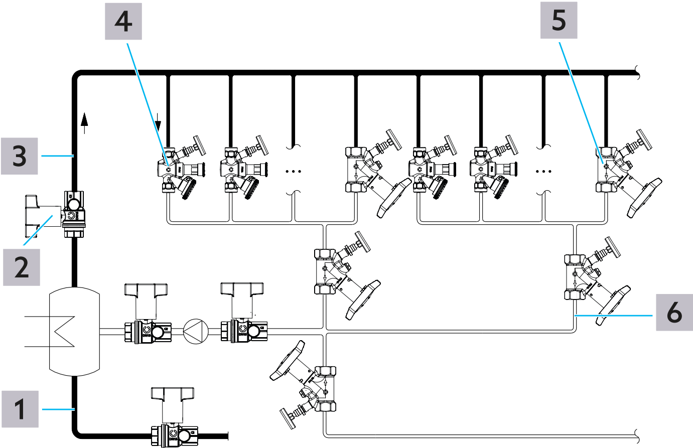
Abb. 4: Anlagenschema
