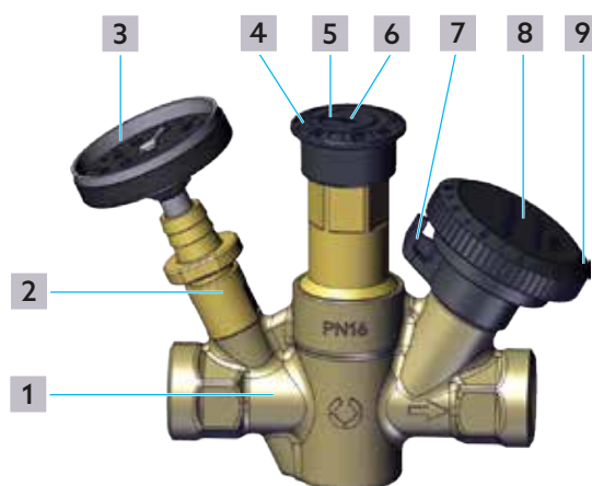
Ryc. 1: Budowa
