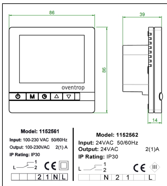
Abb. 4.1 Abmessungen
