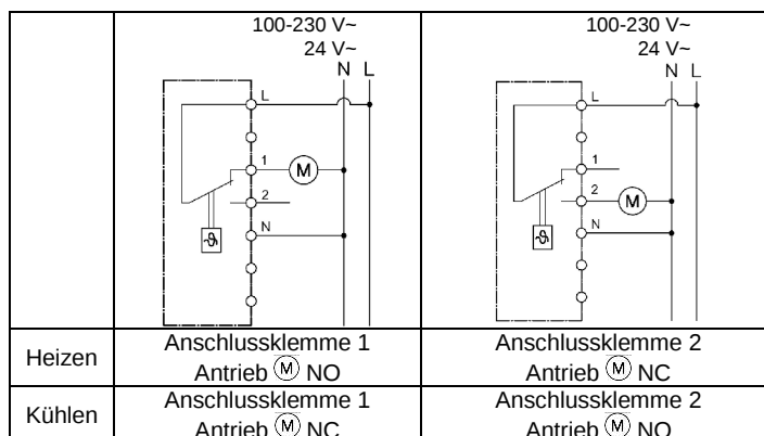
Abb. 6.2 Schaltplan Heizen/Kühlen
