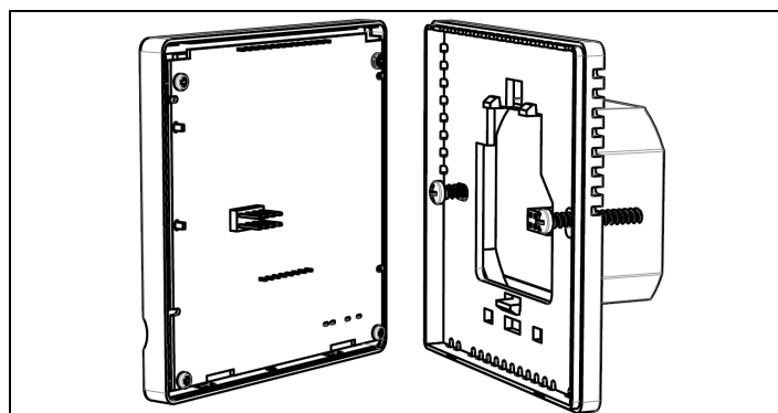
Abb. 6.1 Einbau des Thermostaten
