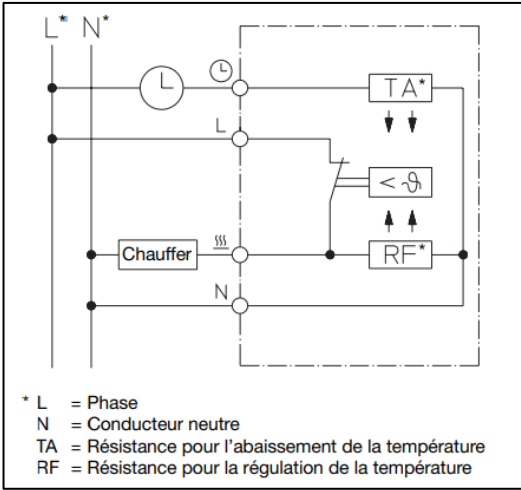
Schéma électrique
