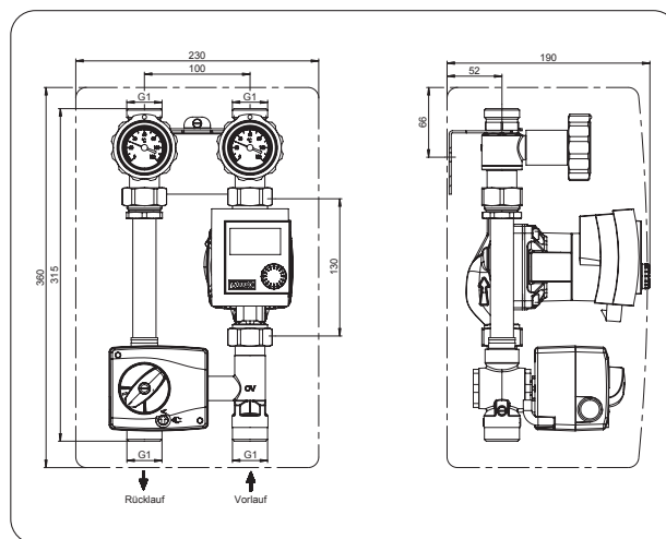
Regumat M3-130
