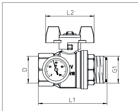
Fig. 4: Dimensions robinet à tournant sphérique en mm
