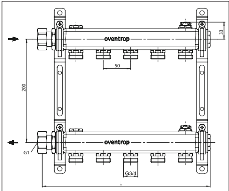
Abb. 2: Maße in mm (Frontansicht)
