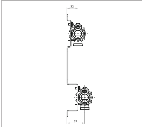
Abb. 3: Maße in mm (Seitenansicht)
