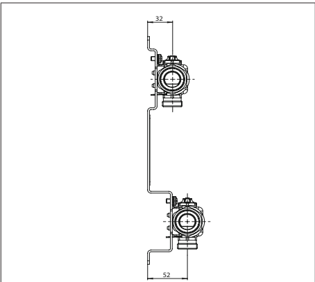
Fig. 3: Dimensions en mm (vue de côté)
