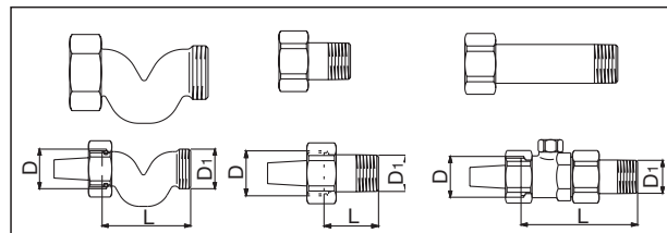
Jeu d'isolation, de compensation et d'arrêt
