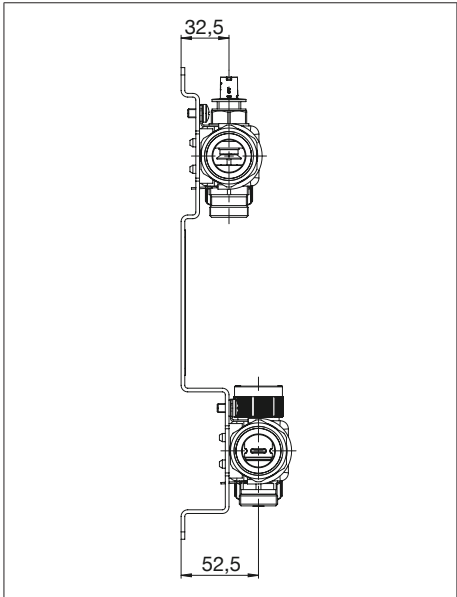
Fig. 7: Encombrements du distributeur/collecteur pour circuits de chauffage Multidis SFQ - vue latérale
