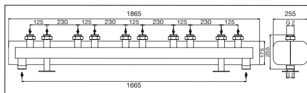
Dimensioni collettore DN 32, 5 circuiti
