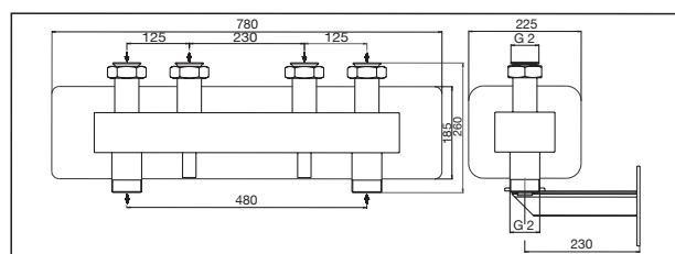
Dimensioni collettore DN 32, 2 circuiti
