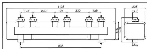
Dimensioni collettore DN 32, 3 circuiti
