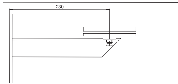
Dimensioni fissaggio a muro per collettore da 4 e 5 circuiti
