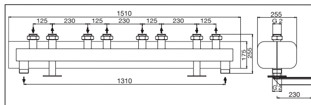
Dimensioni collettore DN 32, 4 circuiti
