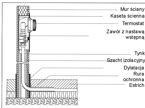
"Unibox E T", głębokość zabudowy 57 mm
