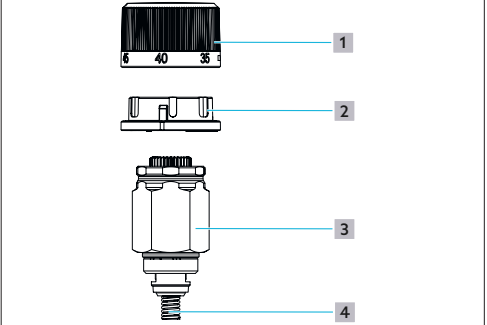
Abb. 1: Aufbau
