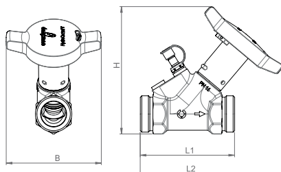
Obr. 3: Rozměry, náhled z boku, vonkajší závit
