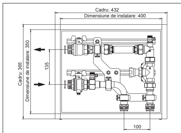
Dimensiuni „Floorbox UH“, racordare orizontală la coloană
