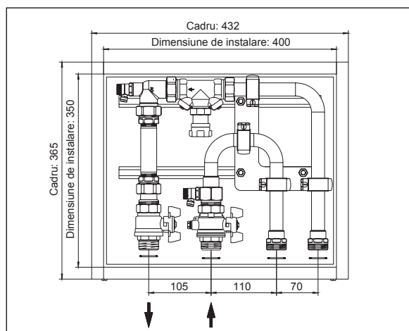
Dimensiuni „Floorbox UV“, racordare verticală la coloană
