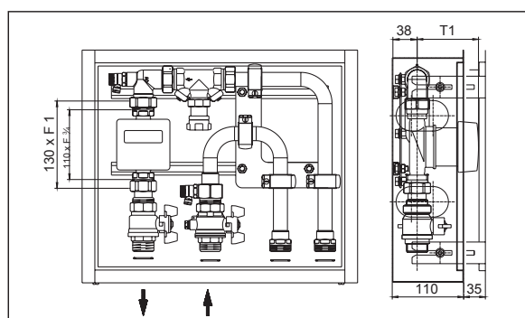
Adâncime de instalare „Floorbox U“
