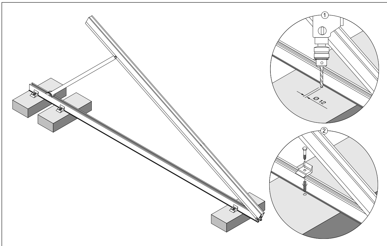
Fig. 25: Fixation des triangles sur support-béton
