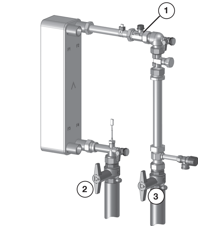
„Sensore di flusso VTH 25“ (cod.art. 1381593); ricambio per stazione produzione ACS „Regumaq X-80“
