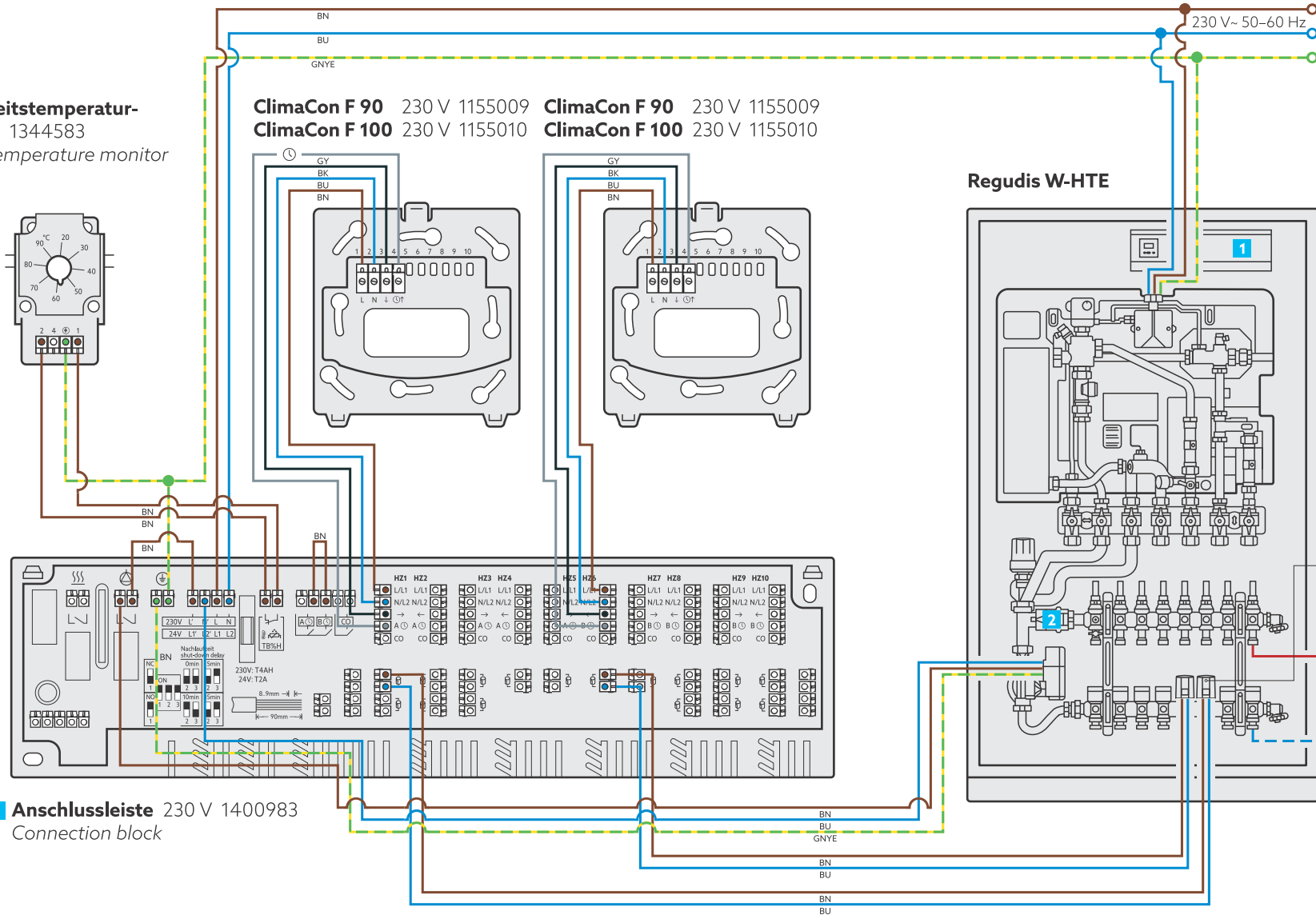
Aktor T 2P 230 V 1012452 (NC) Elektrothermischer Stellantrieb Electrothermal actuator
