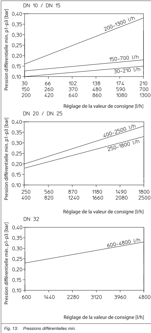
Fig. 13: Pressions différentielles min.
