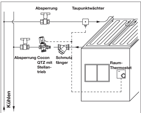
Abb. 6: Einbaubeispiel 1: Zweileitersystem
