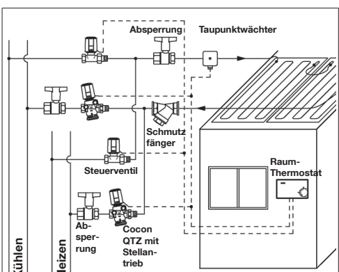
Abb. 7: Einbaubeispiel 2: Vielleitersystem
