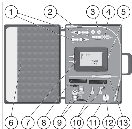
Fig. 1: Leveringsomvang
